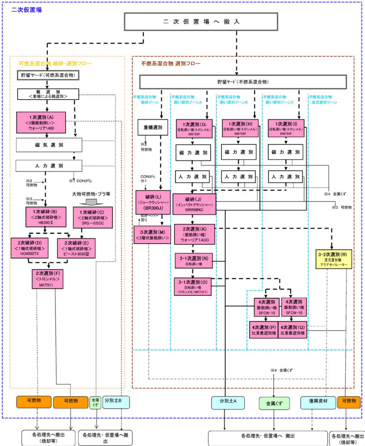
図-2 二次仮置場 全体処理フロー
