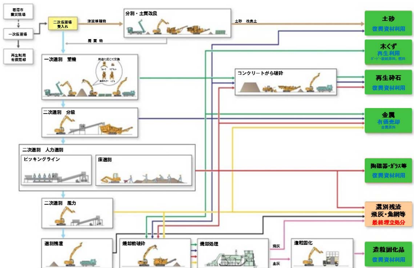
図-4 全体処理フロー図
