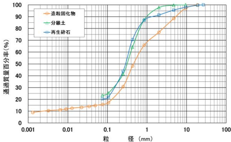
図-9 造粒固化物の材料特性
