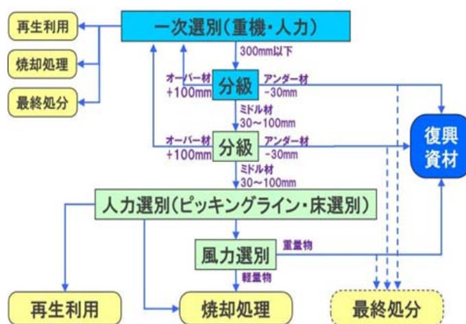
図-6 選別フロー
