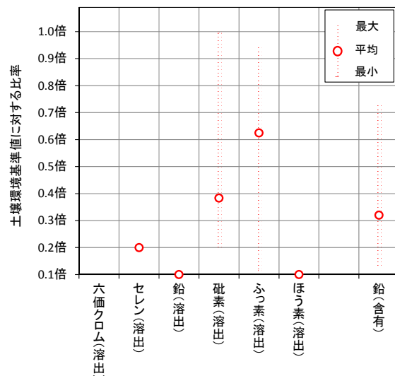
図-13 再生土砂の有害物質分析結果
