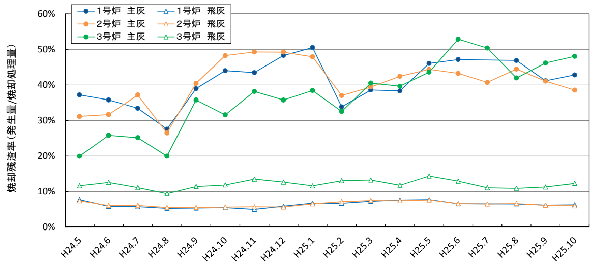
図-8 焼却残渣（主灰・飛灰）の発生率
