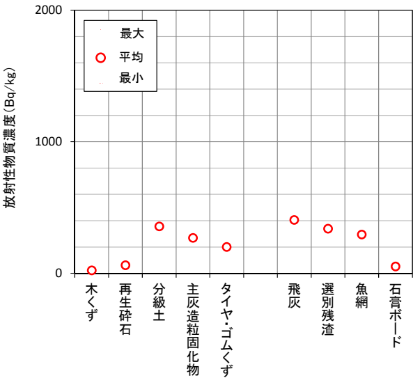
図-10 搬出物の放射性物質濃度
