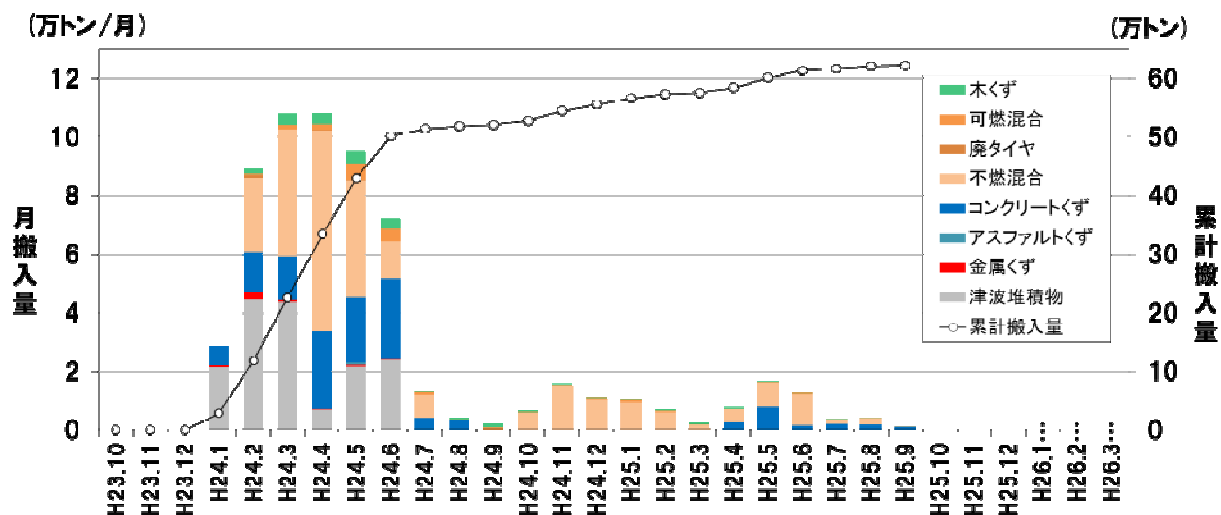
図-5 二次仮置場受入進捗図
