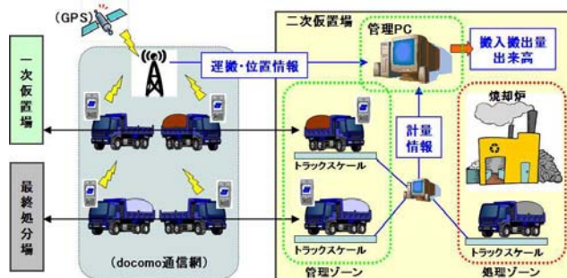
図-14 搬出・搬入管理の概念
