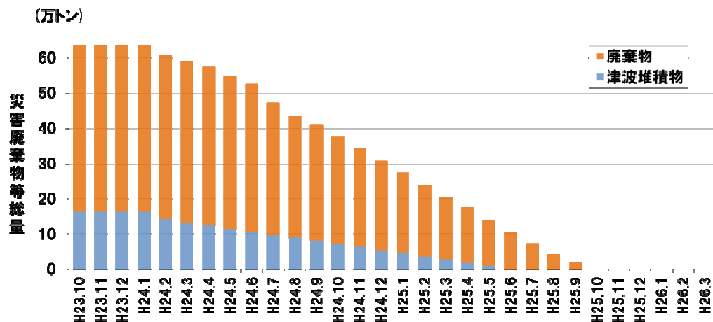
図-3 処理進捗図
