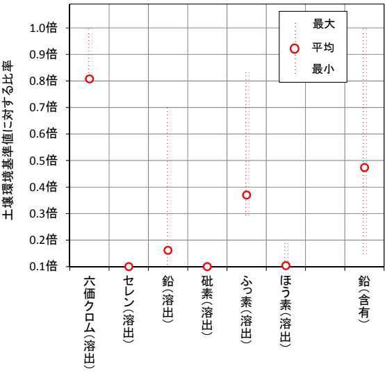
図-11 造粒固化物の有害物質分析
