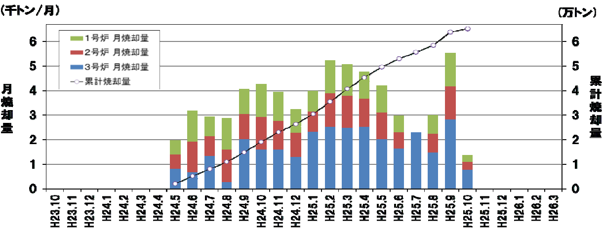
図-7 焼却処理進捗図
