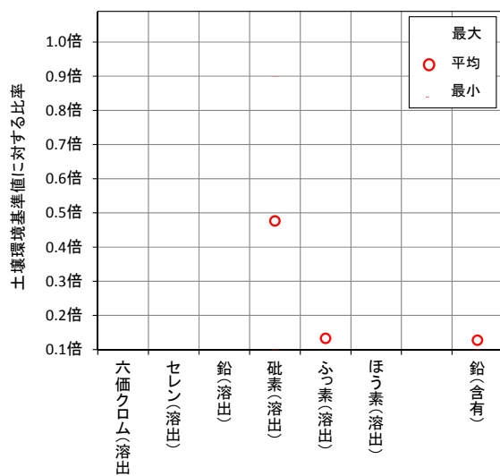
図-12 再生砕石の有害物質分析結果
