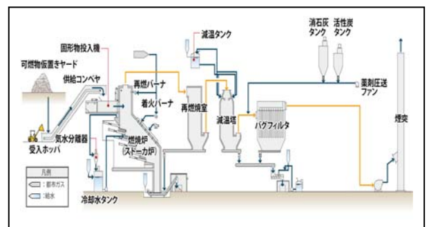
図-4 ストーカ炉 : 110t/日
