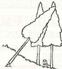
(図3)かかられている立木の伐倒
