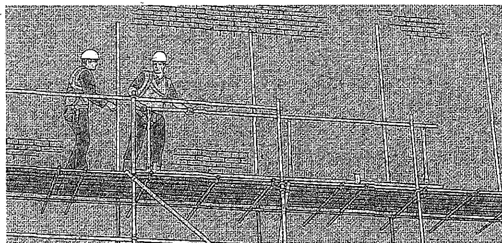
例 2 : 水平方向にスライドする先行手すりわく
