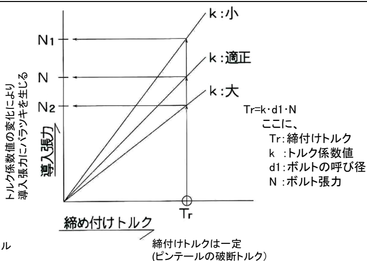
トルシア形高力ボルトの場合
