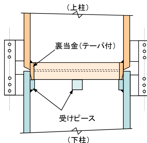
裏当て金が上柱付き
