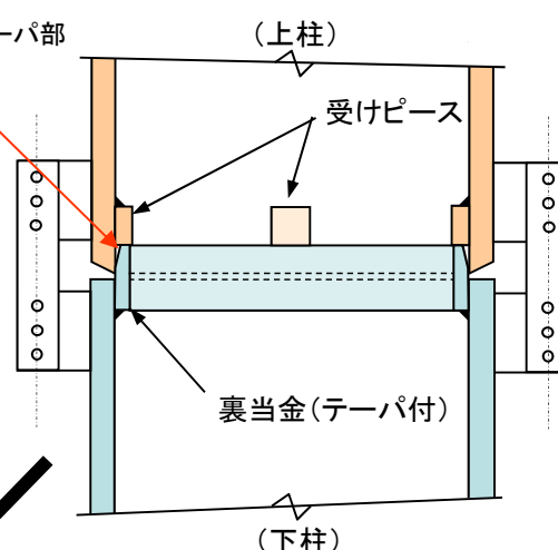
裏当て金が下柱付き
