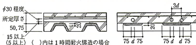
フロアダクト下側のコンクリート厚さが40mm以下の場合
