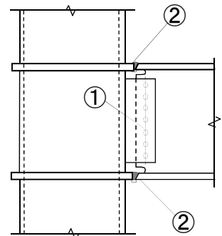
混用接合の姿図
