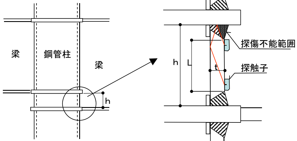
探傷不能範囲概念図
