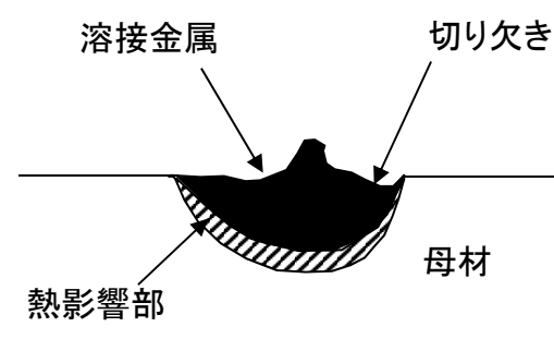
アークストライクの断面例
