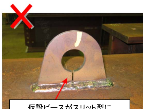
仮設ピースがスリット型になっている
