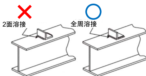
ピース類の溶接
