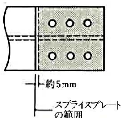
フランジ部
