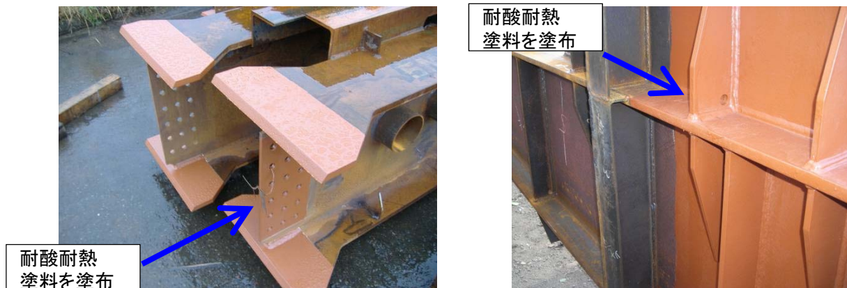
耐酸耐熱塗料の塗布例
