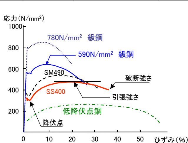
種々の鋼材の応力-ひずみ曲線
