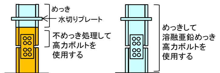
高力ボルト接合部の正しい事例
