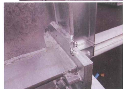
裏当て(めっき後)
