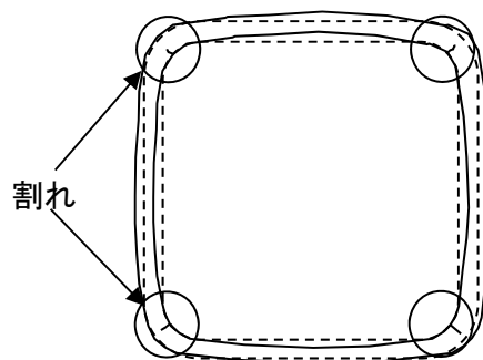
角形鋼管の割れ発生位置 と断面変形想定図
