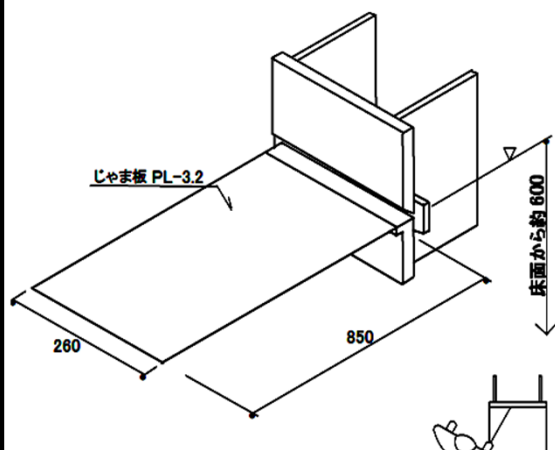
工場溶接
