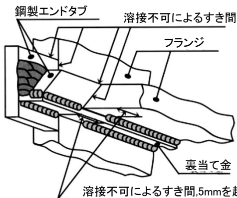
裏当て金・鋼製エンドタブの組立て溶接要領
