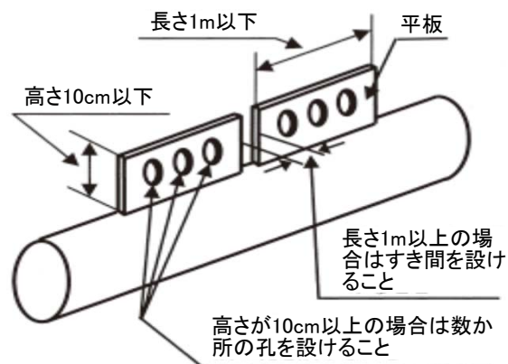
ガセットプレートの取付け要領
