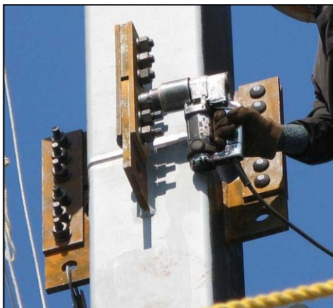
一般的なエレクションピース
