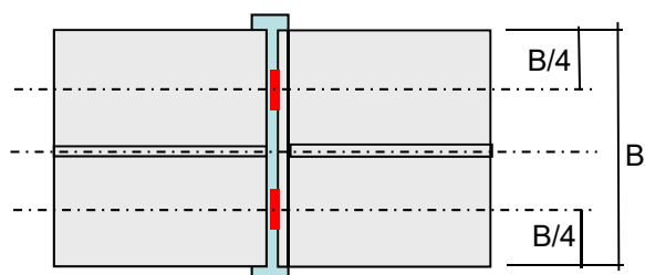
開先内での組立て溶接:OK
