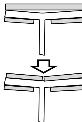
外側のスプライスプレート も2枚に割る
