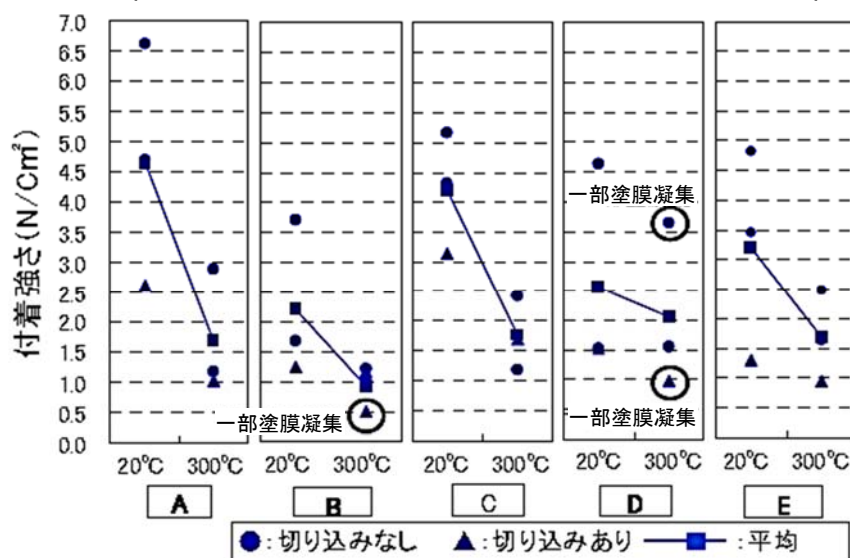
半乾式吹付岩綿の付着力試験結果
