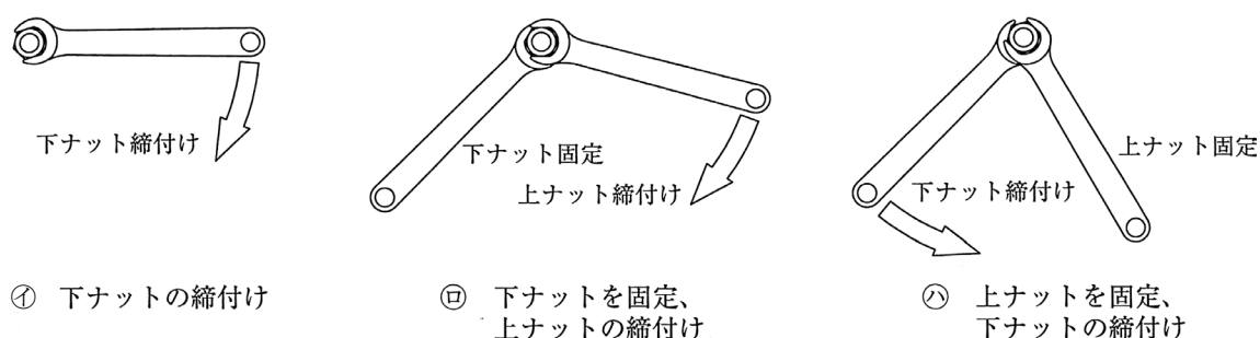
二重ナットの締付け
