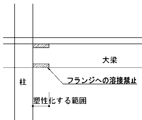
(a) 梁端部の金物溶接禁止位置
