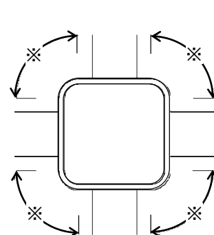
(c) 冷間成形角形鋼管柱の角部
