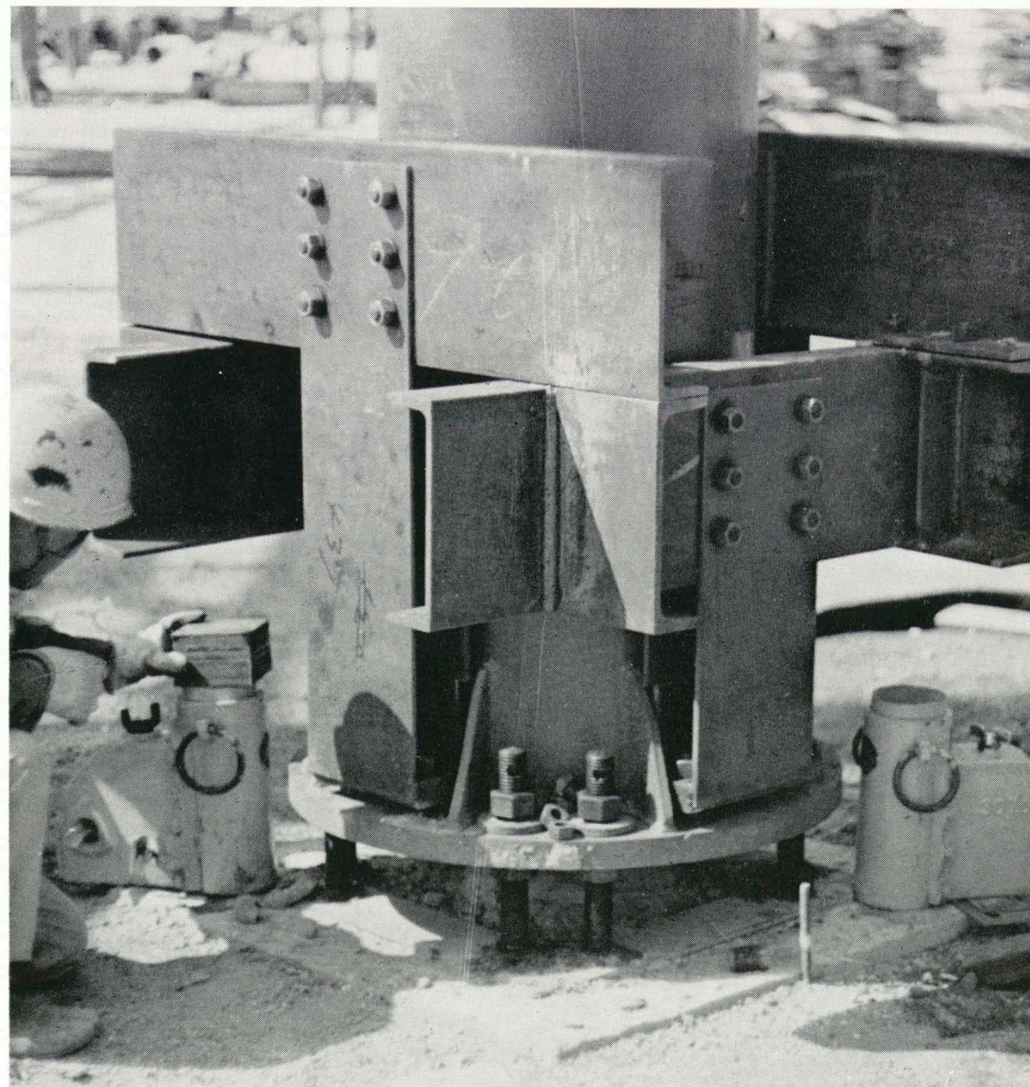
かさ上げ工法 'Living leg' Adjustable column
