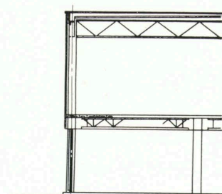
断面
