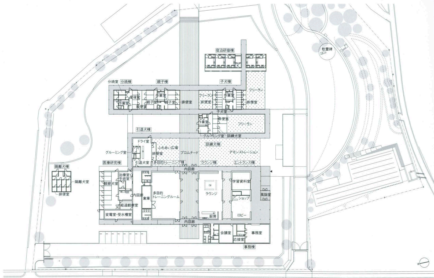
1階平面 縮尺1/1,000
