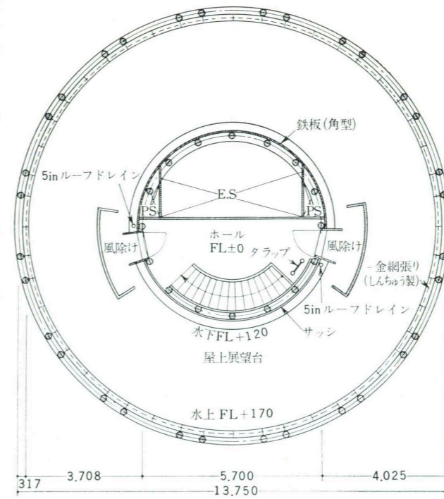
(a) 屋上展望台 S.G.L.+90.240 (ホール床) 収容人員 180人
