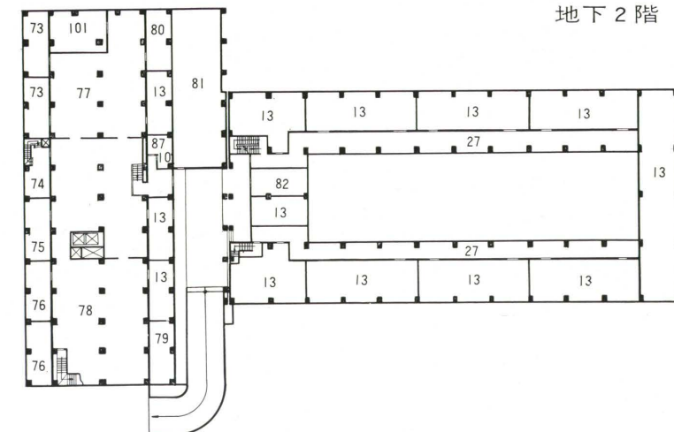
地下2階
