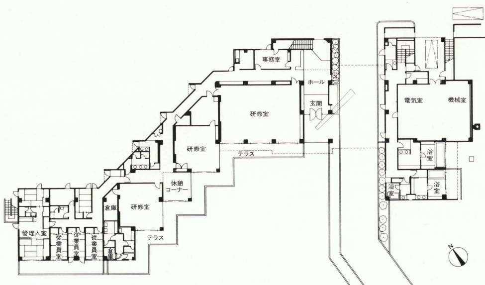
1 階平面
