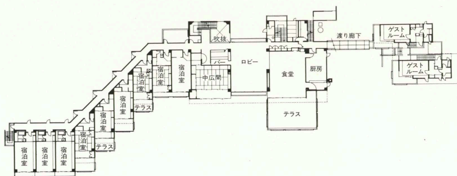
2 階平面
