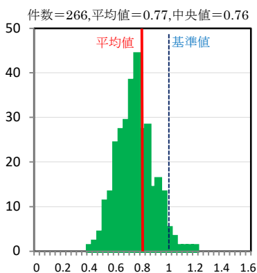
図5 BPI 値分布図
