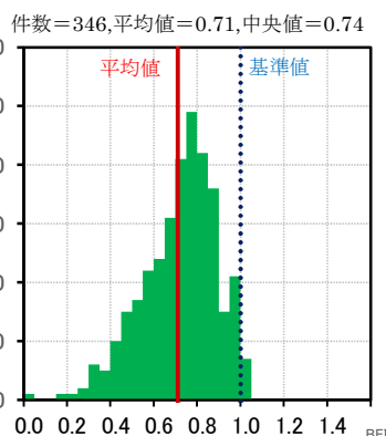
図6 BEI 値分布図 (非住宅)
