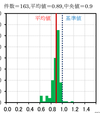
図7 BEI 値分布図 (集合住宅)
