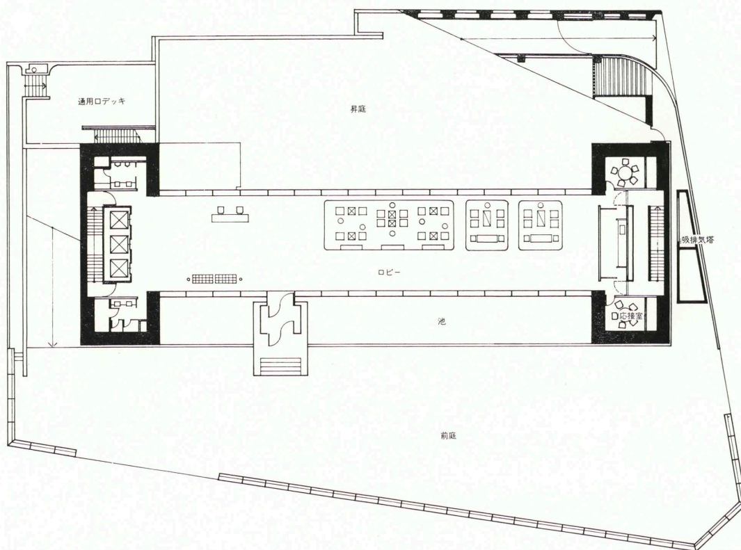
1階平面図
