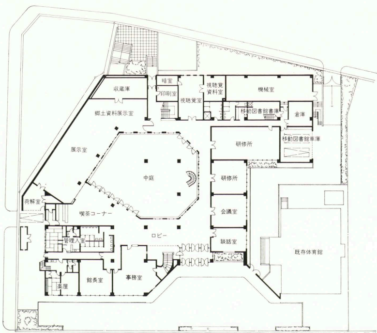
1階平面図
