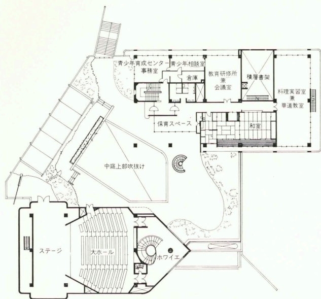
2階平面図
