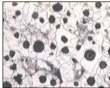
ダクタイル鑄鉄 ( F C D 4 5 0 )
