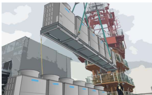
【空調機・架台一体化揚重】
