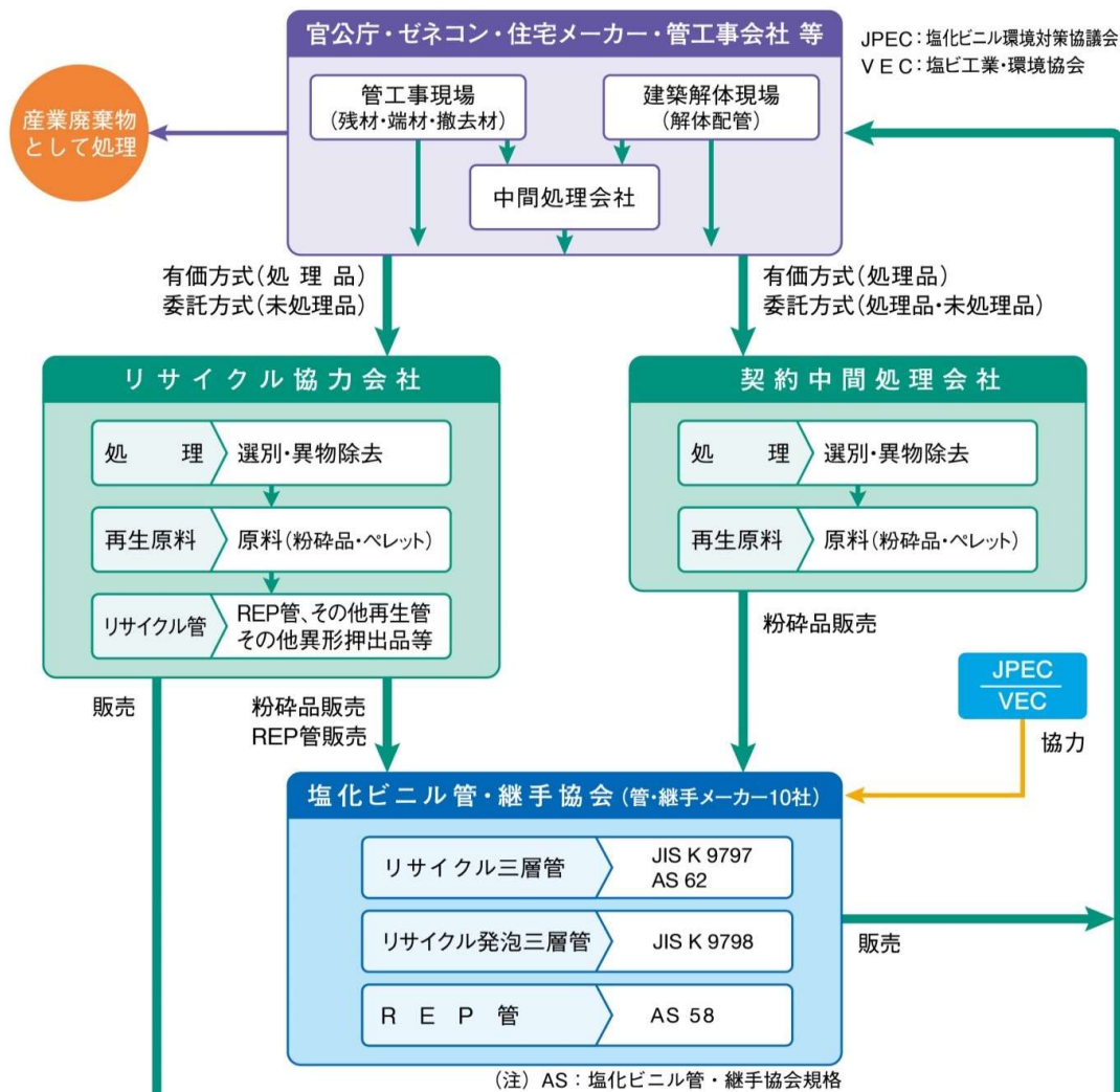
■ マテリアルリサイクルシステム図
