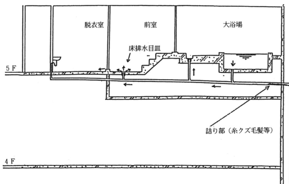
図-1 大浴室の排水ルート（断面）
