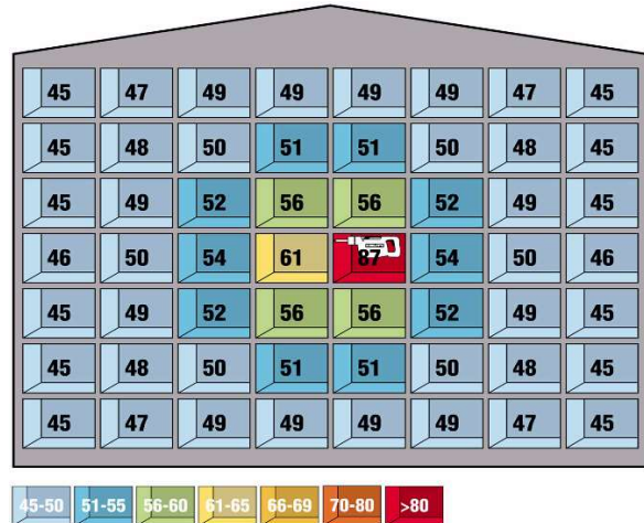
低騒音型ドリル (DD30-W)
