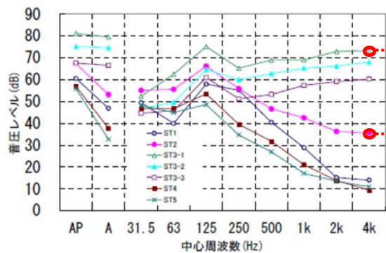
低騒音ドリルM10の騒音
