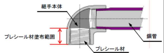
シール材付ねじ込み式継手（断面）
