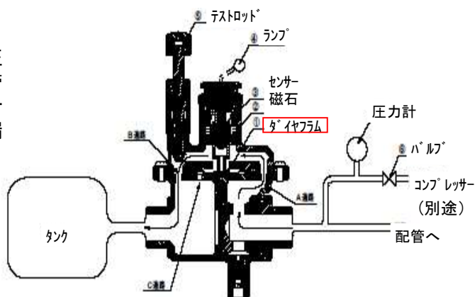
HWR-301用センサー本体の構造
