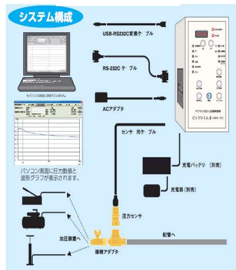
HWR-701のシステム構成
