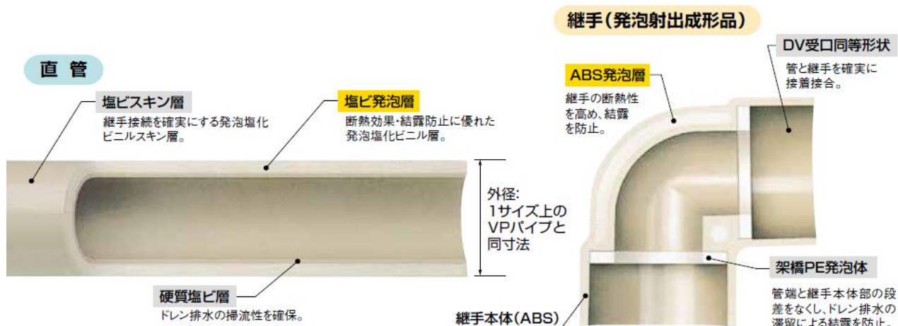
ACドレンパイプ、継手の構造
