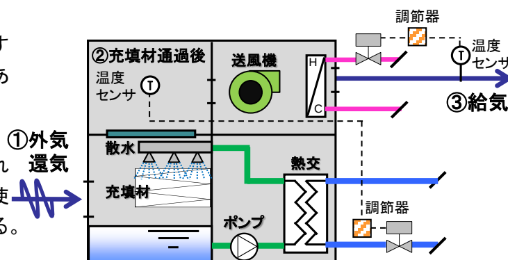
図2 制御概要図
