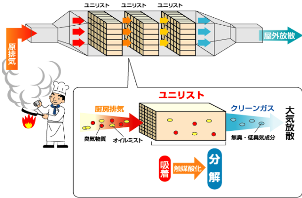
脱臭のメカニズム
