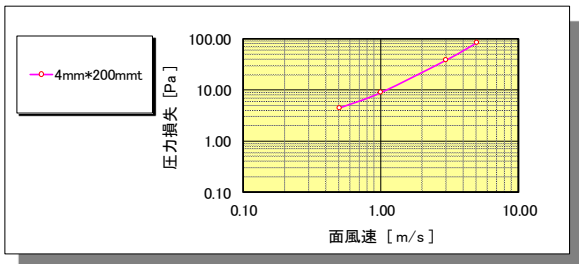
圧力損失カーブ
