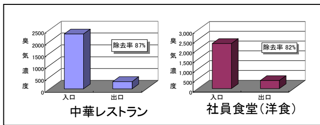
図-1 現地試験評価結果
