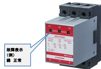
SPDの故障表示例
