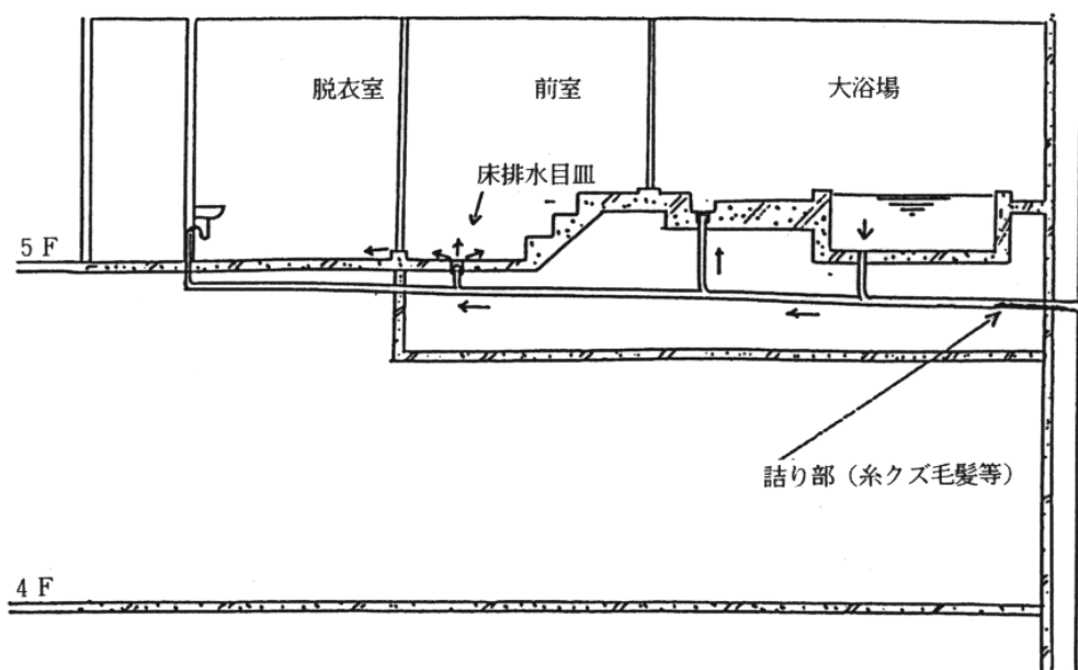
図-1 大浴室の排水ルート（断面）
