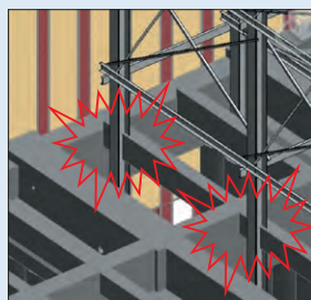
干渉箇所の課題抽出① 構台杭ー梁干渉
