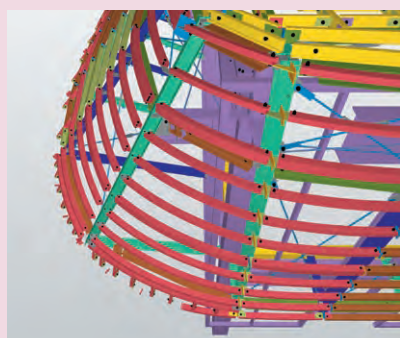
屋根／鉄骨下地の湾曲部納まり検討
