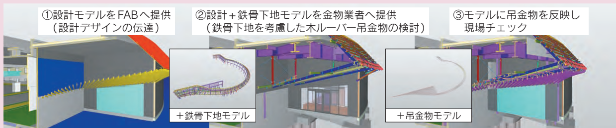
専門工事会社とのデータ連携(設計デザインを鉄骨下地に反映、鉄骨下地をふまえて吊金物を検討と段階的に連携)
