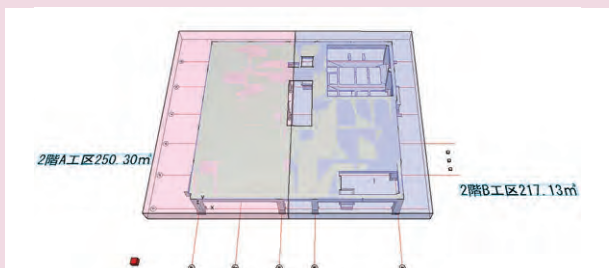
コンクリート打設数量の算出を行い、打継検討に活用
