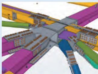
鉄骨仕口詳細
