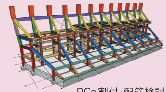
PCa割付・配筋検討
