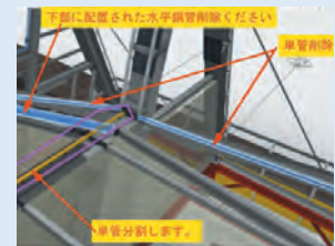
下地単管の納まり検討
