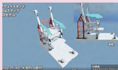
4D(動画)による見える化(PCa)
