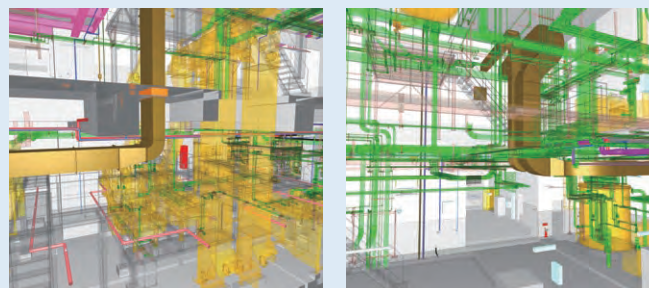
Rebroでの空間調整・干渉チェック (BIMユーザー)
