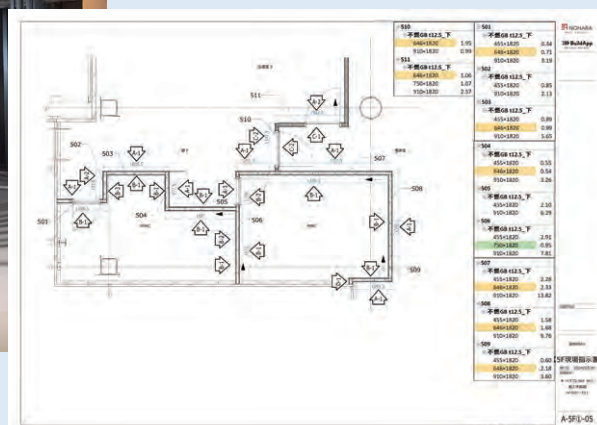
施工状況とボード割付図
