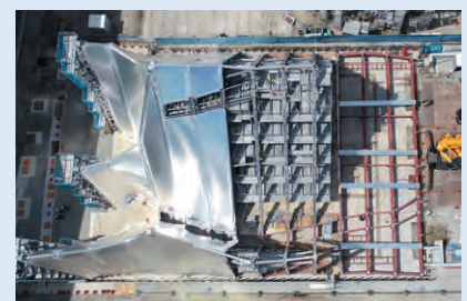
外装膜の施工状況
