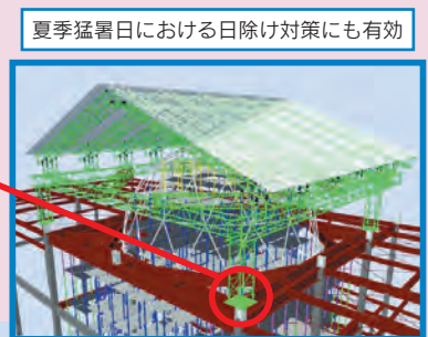
仮設屋根と本体鉄骨柱との関係
