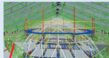
仮設屋根からの吊り足場設置計画
