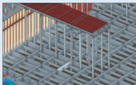
概略モデルでの検討完了 構台杭と構造躯体の位置調整
