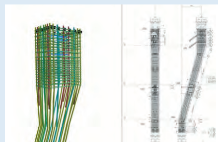
配筋の納まり検討 (Archicad、3D AutoCAD)
