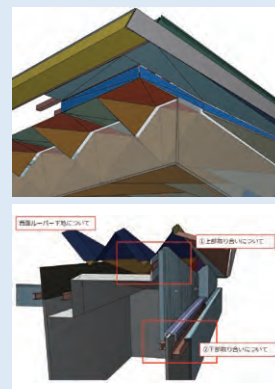
取合い納まり確認
