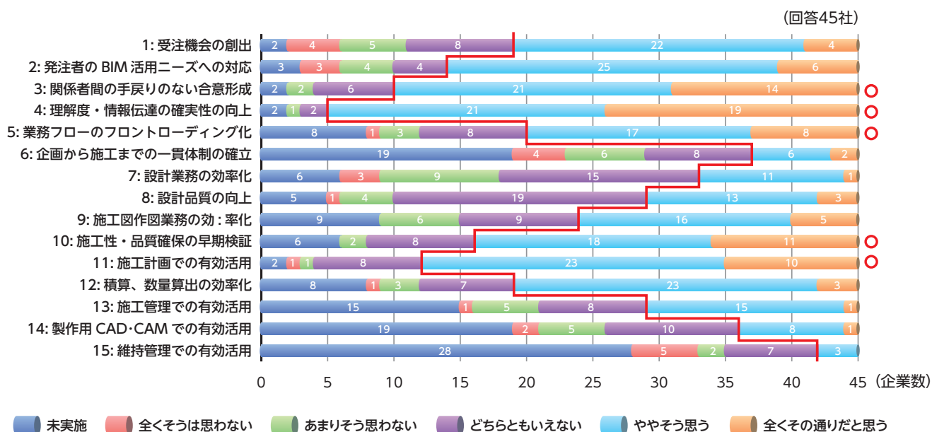
図28 BIMの効果
