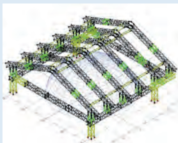
仮設屋根アイソメ図
