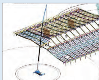
一番負荷がかかる箇所、 干渉の恐れがある箇所で検証
