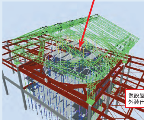
仮設屋根と建築BIMモデルとの合成
