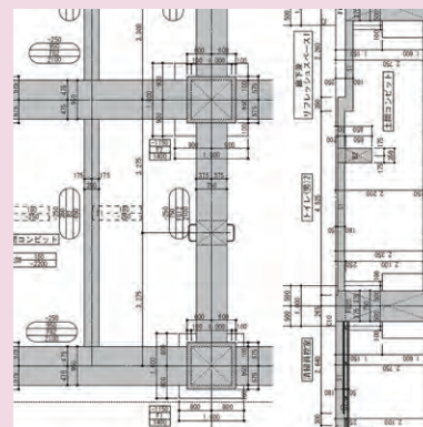
2DCADに落とし込んで 早期に一次躯体図を作成
