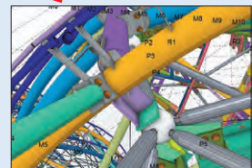
アンモナイト棟： 下部トラスとのジョイント例
