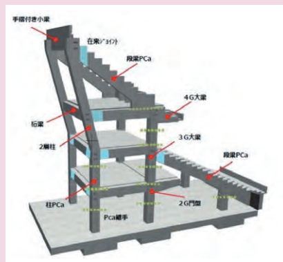
PCa部材の割付検討
