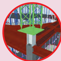
仮設屋根と本体鉄骨柱との関係
