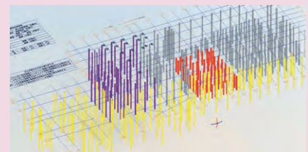
出来高モデル
