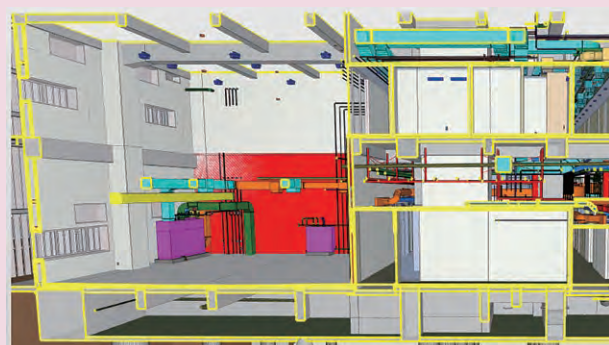
構造躯体と設備配管の可視化で干渉を確認
