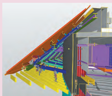
外壁／ACW／鉄骨貫通部の納まり検討
