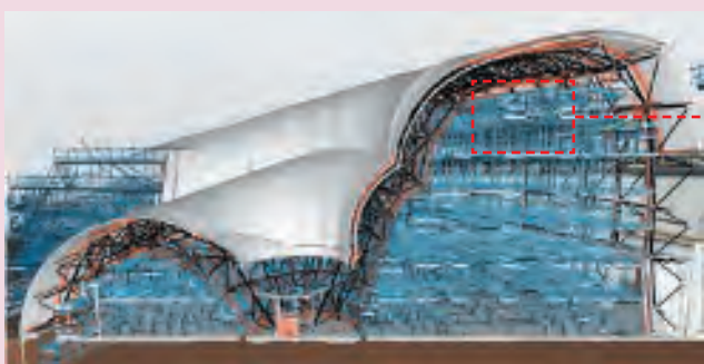
支保工を統合した BIM モデル
