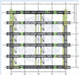
仮設屋根アイソメ図
