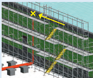
&lt;足場計画初期段階&gt;
