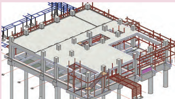
増し打ち箇所など可能な限り詳細な建築モデルを作成
