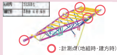
屋根鉄骨ユニット形状
