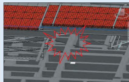
干渉箇所の課題抽出② プレスー梁干渉
