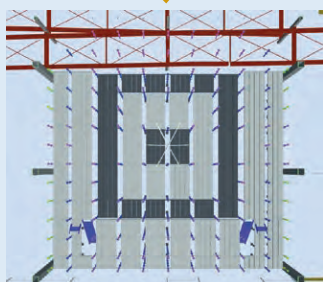
足場建地割付平面図
