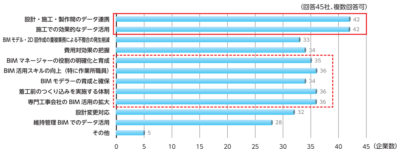
図29 BIMの課題
