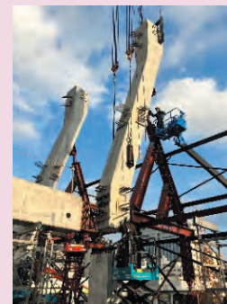
大型PCa揚重状況
