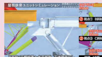
4D(動画)による見える化(屋根鉄骨)
