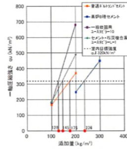
図-10 各種固化材の一軸圧縮強度結果(α25)
