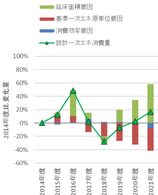
図Ⅲ-2-21 設計一次エネルギー消費量の2014年度比推移と増減要因分析
