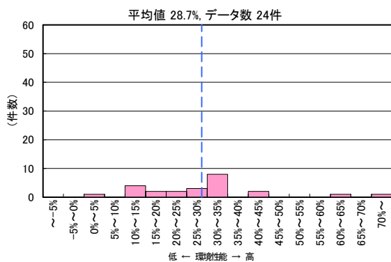
図Ⅱ-2-82 CASBEE 評価 LCCO 2 低減率の分布 2021度 非住宅（標準入力法等）
