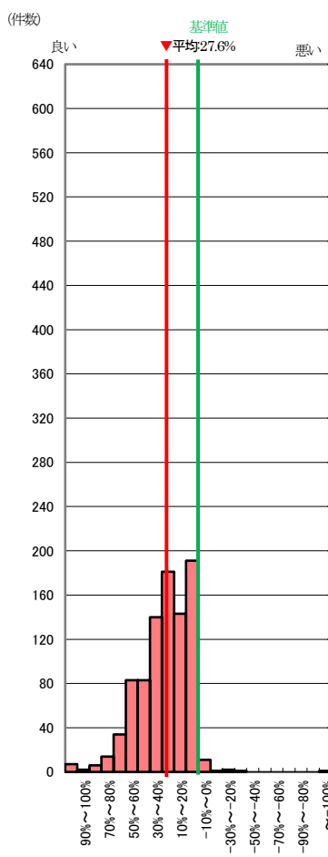
図 II-1-10 2013～2021 年度 BEI 値 建物全体基準値からの削減
