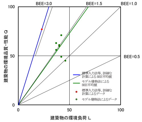
図II-2-31 CASBEE 評価 BEE 値プロット図 (2021 年度 学校)
