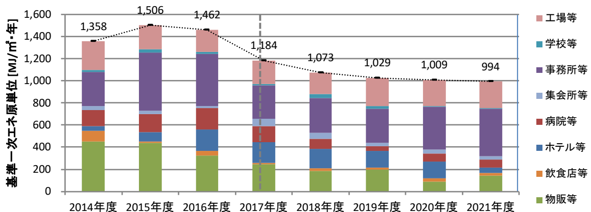
図Ⅲ-2-19 2014 年度以降の全体の基準一次エネ原単位の建物用途内訳
