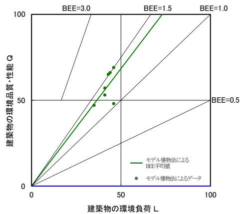
図II-2-32 CASBEE 評価 BEE 値プロット図 (2020 年度 物販店)
