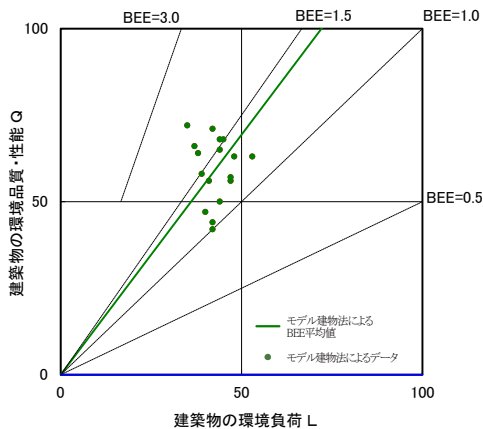
図II-2-39 CASBEE 評価 BEE 値プロット図 (2020 年度 病院)
