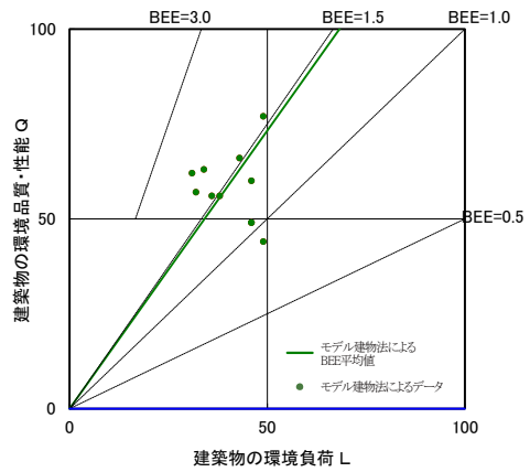
図II-2-42 CASBEE 評価 BEE 値プロット図 (2021 年度 ホテル)
