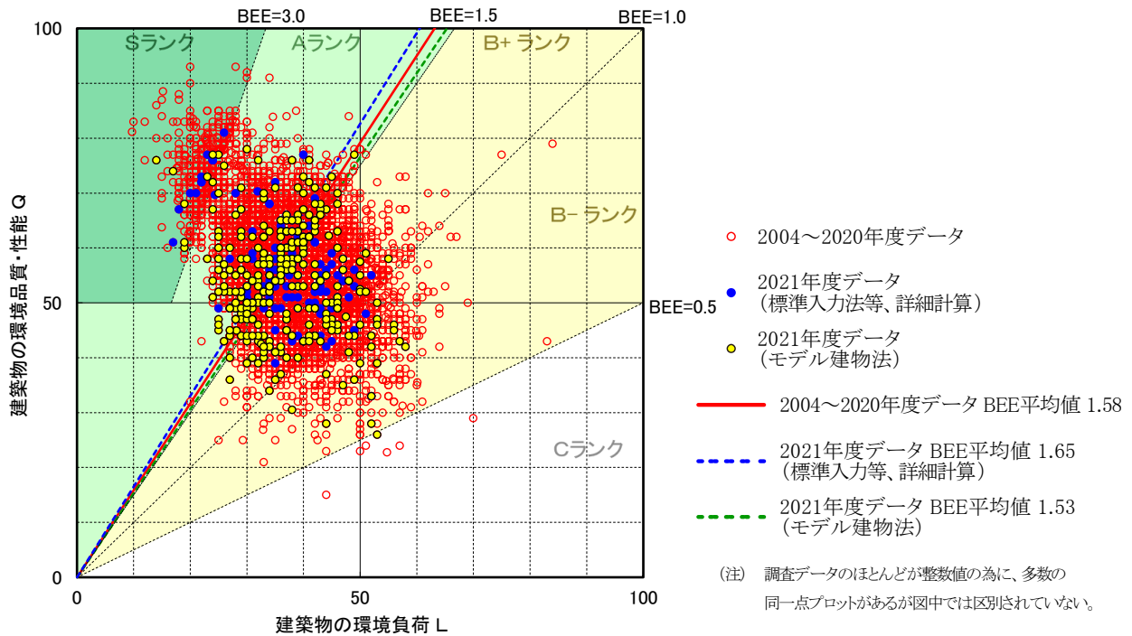
図II-2-47 CASBEE評価 BEE 値プロット図 (2004～2021年度データ 全用途)
