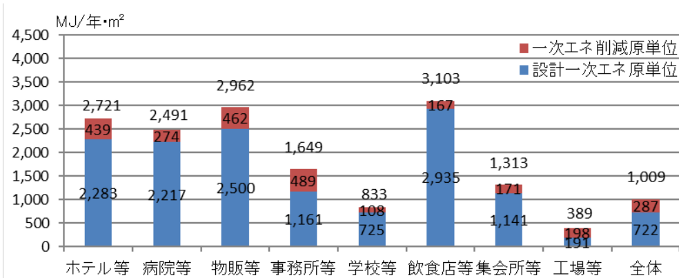
図Ⅲ-2-6 建物用途毎の設計一次エネ原単位と一次エネ削減原単位（前年度調査分）
