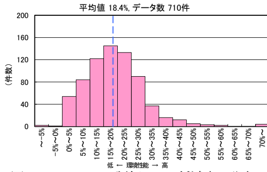
図 II-2-84 CASBEE 評価 LCCO 2 低減率の分布 (2008 年度～2020 年度 事務所)
