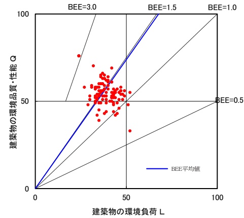
図II-2-44 CASBEE 評価 BEE 値プロット図 (2021 年度 集合住宅)
