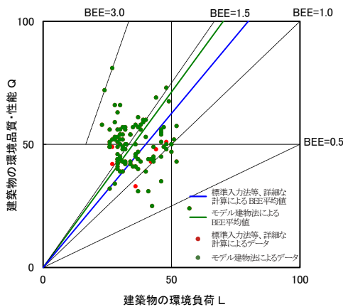
図II-2-37 CASBEE 評価 BEE 値プロット図 (2020 年度 工場)
