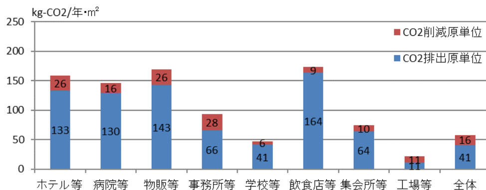
図Ⅲ-2-8 建物用途毎のCO 2 排出原単位とCO 2 削減原単位（前年度調査分）
