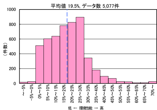
図Ⅱ-2-78 CASBEE評価 LCCO 2 低減率の分布 全用途（2008年度～2020年度）
