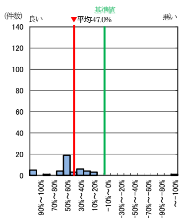
図 II-1-9 2021 年度 BEI 値 建物全体基準値からの削減
