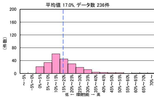
図 II-2-87 CASBEE 評価 LCCO 2 低減率の分布 (2008 年度～2020 年度 学校)
