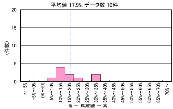
図II-2-103 CASBEE 評価 LCCO 2 低減率の分布 (2021年度 ホテル モデル建物法)
