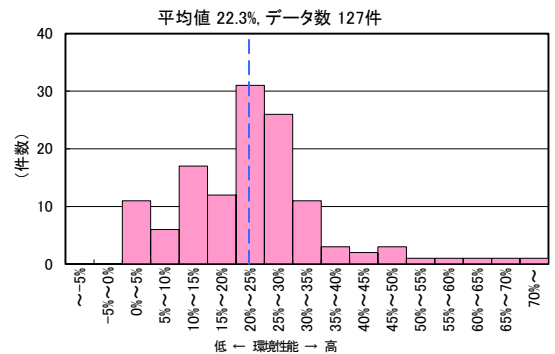
図 II-2-98 CASBEE 評価 LCCO 2 低減率の分布 (2021 年度 工場 モデル建物法)
