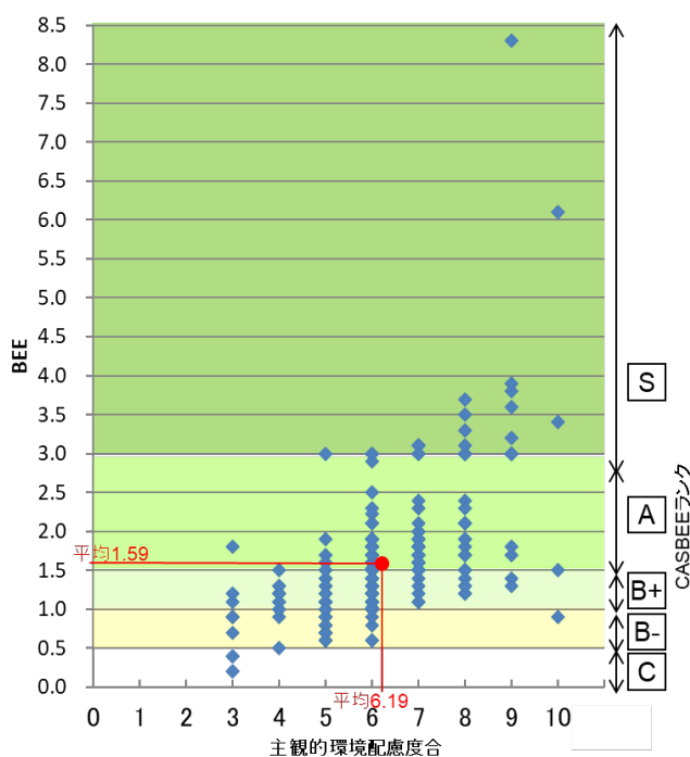
図Ⅱ-2-100 主観的環境配慮度合と BEE の度数分布(2021 年度) (N=291)
