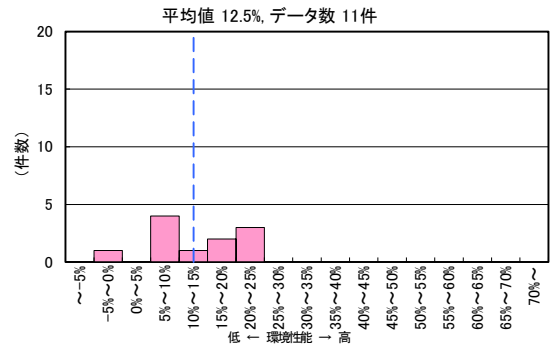
図 II-2-101 CASBEE 評価 LCCO 2 低減率の分布 (2021 年度 病院 モデル建物法)
