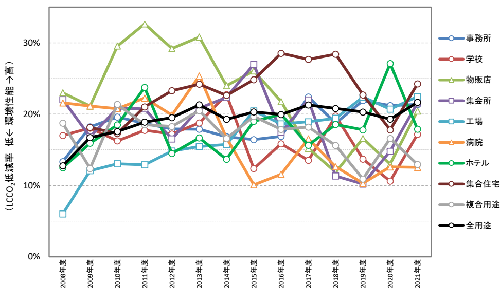
図II-2-75 CASBEE 評価におけるLCCO 2 低減率の建物用途別平均値 (2008年度～2021年度データ)
