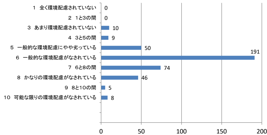
図Ⅱ-2-104 主観的環境配慮度合の度数分布 (2021 年度) (N=393)
