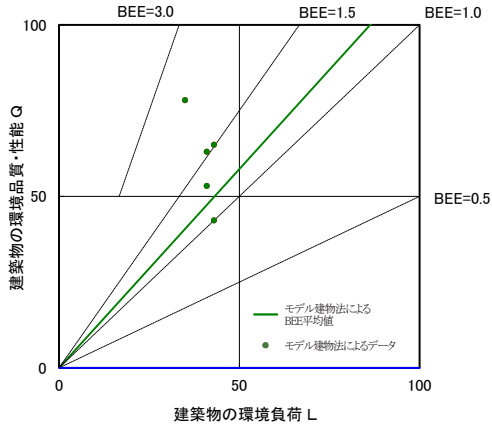
図II-2-30 CASBEE 評価 BEE 値プロット図 (2020 年度 学校)
