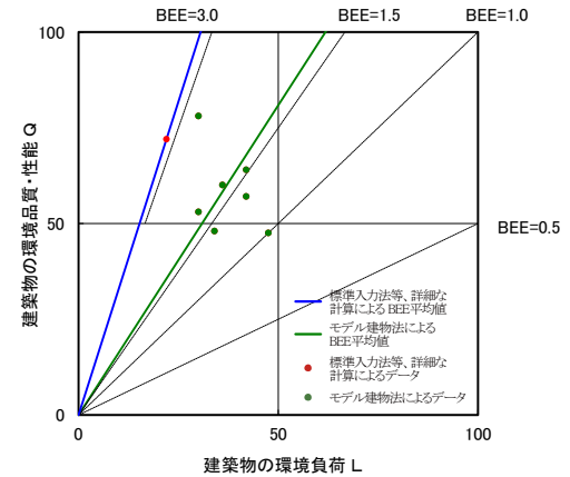
図II-2-33 CASBEE 評価 BEE 値プロット図 (2021 年度 物販店)
