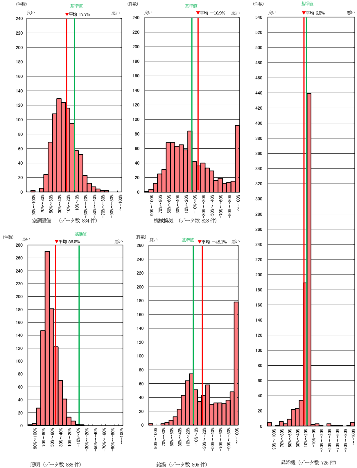
図Ⅱ-1-13 2013～2021年度 標準入力法 各設備機器 基準値からの削減率
