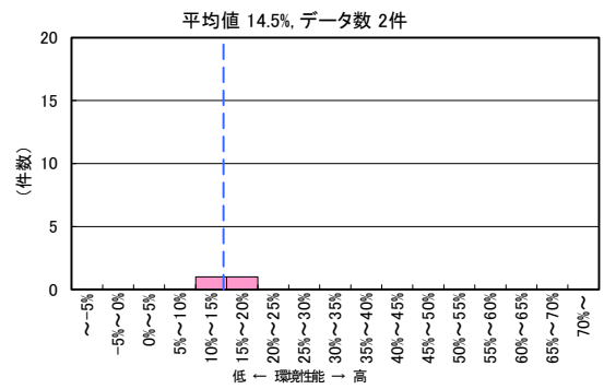
図II-2-105 CASBEE 評価 LCCO 2 低減率の分布 (2021年度 複合用途 標準入力法等)
