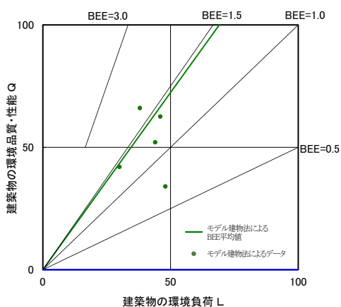
図II-2-35 CASBEE 評価 BEE 値プロット図 (2020 年度 集会所)
