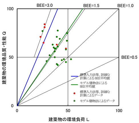
図II-2-45 CASBEE 評価 BEE 値プロット図 (2020 年度 複合用途)
