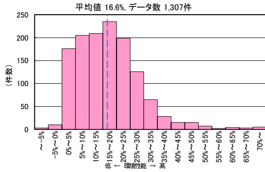
図 II-2-96 CASBEE 評価 LCCO 2 低減率の分布 (2008 年度~2020 年度 工場)
