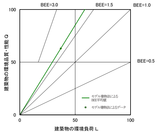
図II-2-34 CASBEE 評価 BEE 値プロット図 (2021 年度 飲食店)
