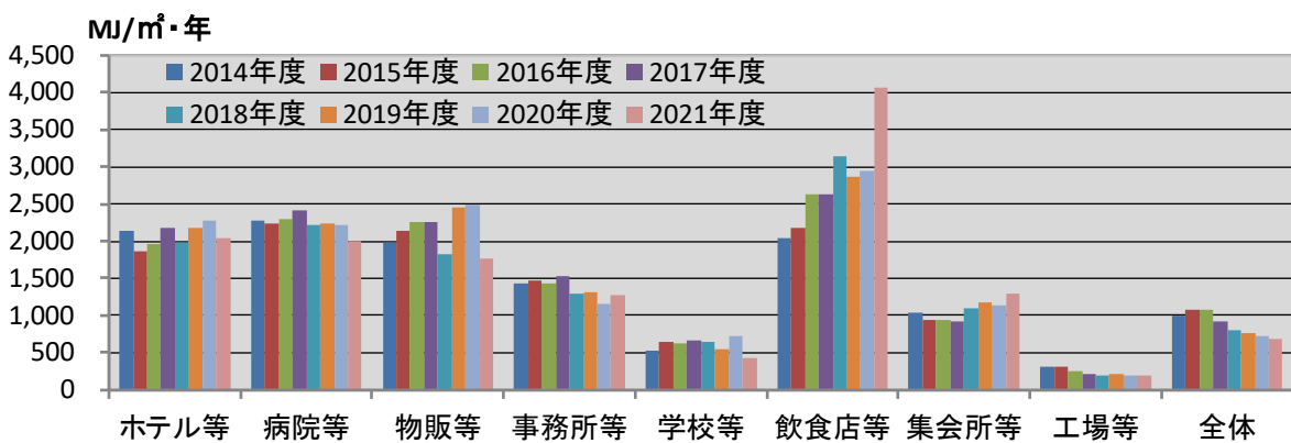
図Ⅲ-2-13 2014 年度以降の建物用途毎 設計一次エネ原単位の推移
