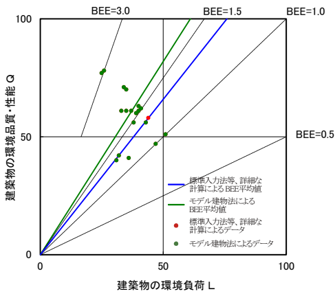
図II-2-41 CASBEE 評価 BEE 値プロット図 (2020 年度 ホテル)
