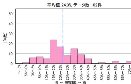
図Ⅱ-2-81 CASBEE 評価 LCCO 2 低減率の分布 (2021年度 集合住宅)
