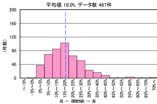
図II-2-104 CASBEE 評価 LCCO 2 低減率の分布 (2008年度~2020年度 複合用途)
