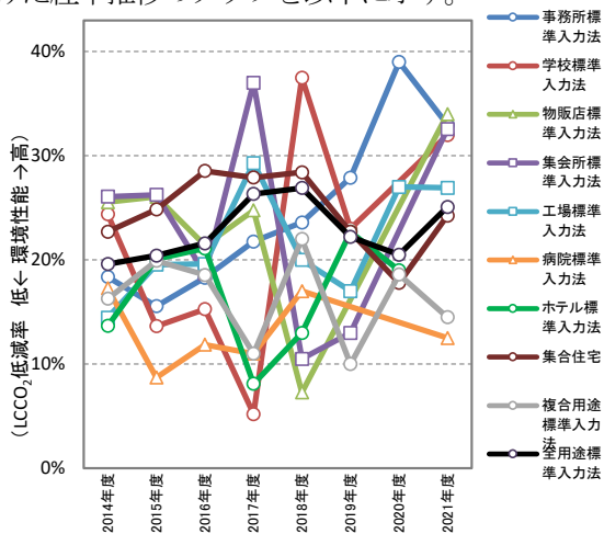
図II-2-76 CASBEE 評価におけるLCCO 2 低減率の建物用途別平均値 (標準入力法等 2014年度～2021年度)
