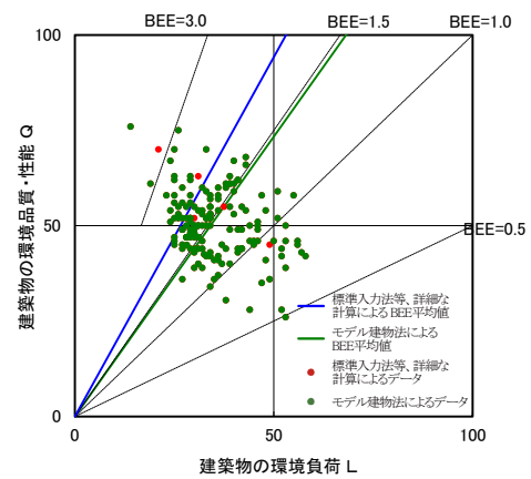
図II-2-38 CASBEE 評価 BEE 値プロット図 (2021 年度 工場)
