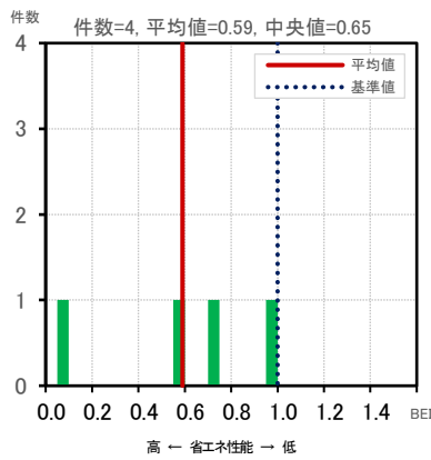
図II-1-31 BEIの分布 (飲食店等 モデル建物法)
