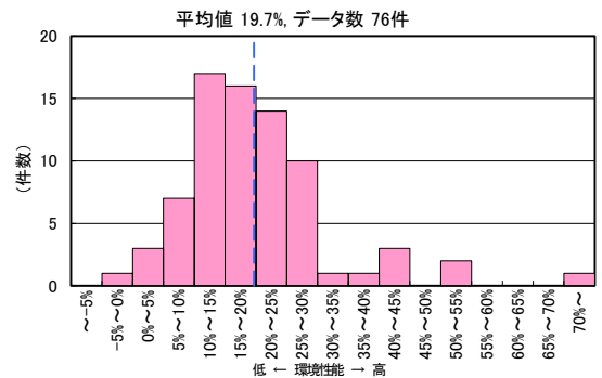
図 II-2-86 CASBEE 評価 LCCO 2 低減率の分布 (2021 年度 事務所 モデル建物法)
