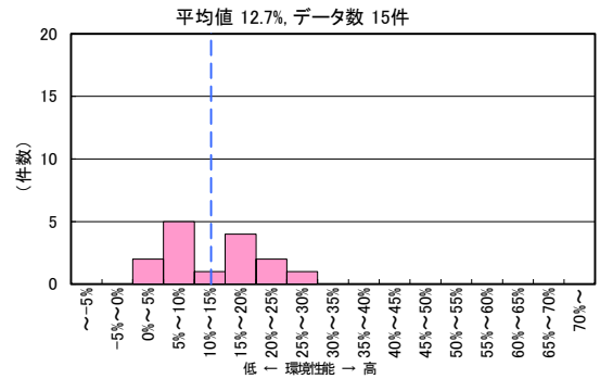
図II-2-106 CASBEE 評価 LCCO 2 低減率の分布 (2021年度 複合用途 モデル建物法)
