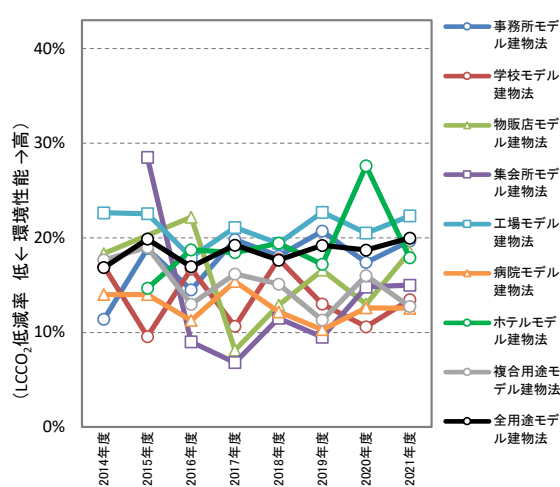
図II-2-77 CASBEE 評価におけるLCCO 2 低減率の建物用途別平均値 (モデル建物法 2014年度～2021年度)
