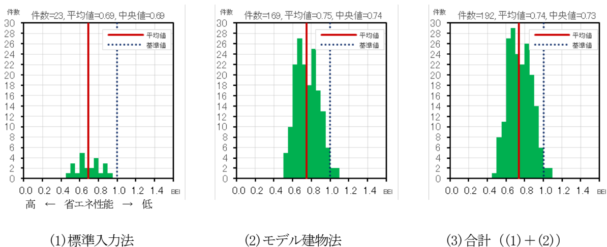
図Ⅱ-1-16 BPI の分布 (事務所)
