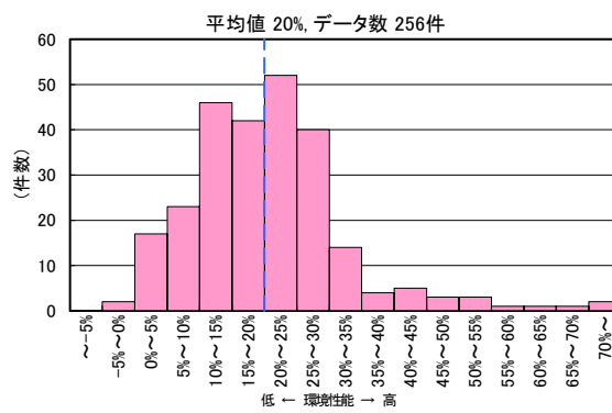
図Ⅱ-2-83 CASBEE 評価 LCCO 2 低減率の分布 2021度 非住宅（モデル建物法）
