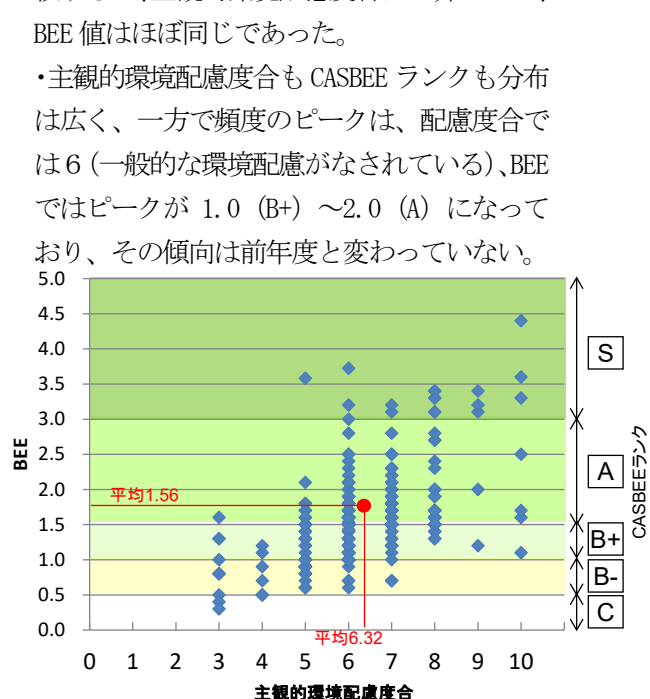
図Ⅱ-2-101 主観的環境配慮度合と BEE の度数分布(2022 年度) (N=353)
