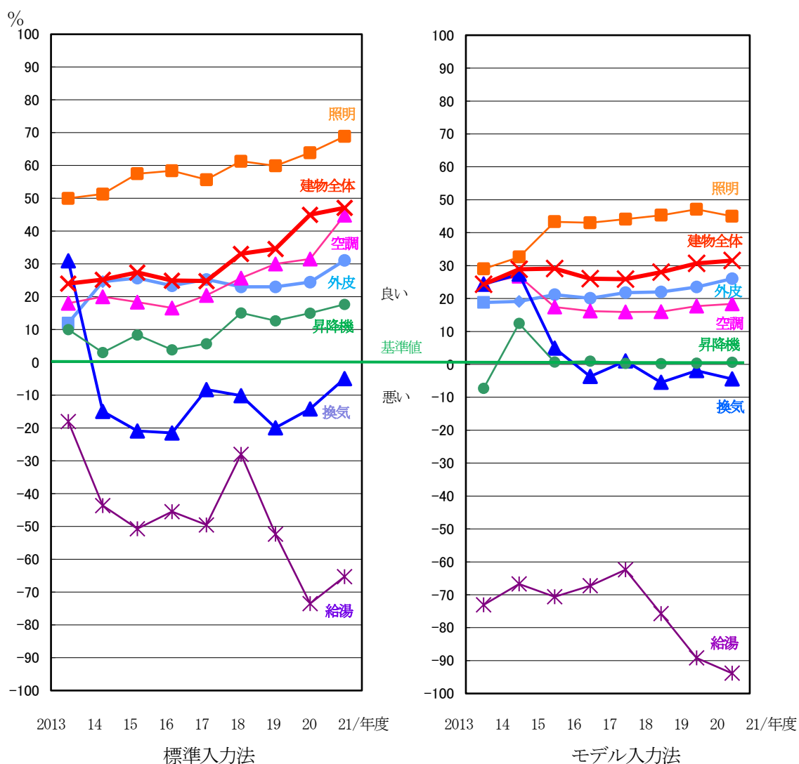
図Ⅱ-1-6 各指標の基準値に対する削減率平均値の推移（2013年度～2021年度）
