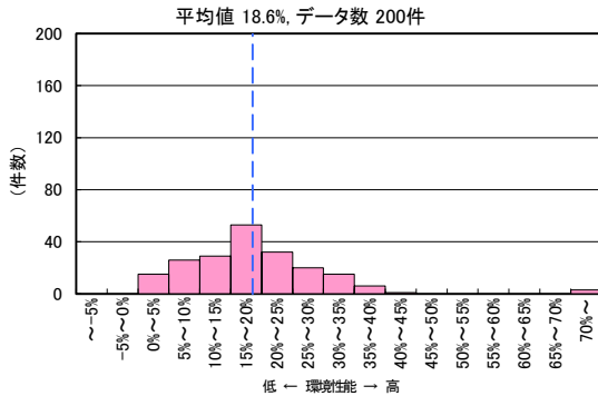
図II-2-102 CASBEE 評価 LCCO 2 低減率の分布 (2008年度~2020年度 ホテル)
