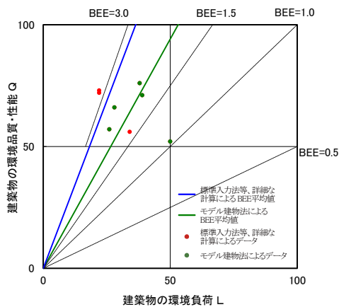
図II-2-36 CASBEE 評価 BEE 値プロット図 (2021 年度 集会所)
