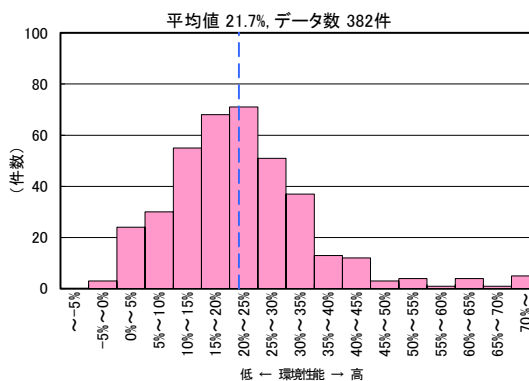
図Ⅱ-2-79 CASBEE評価 LCCO 2 低減率の分布 全用途（2021年度）
