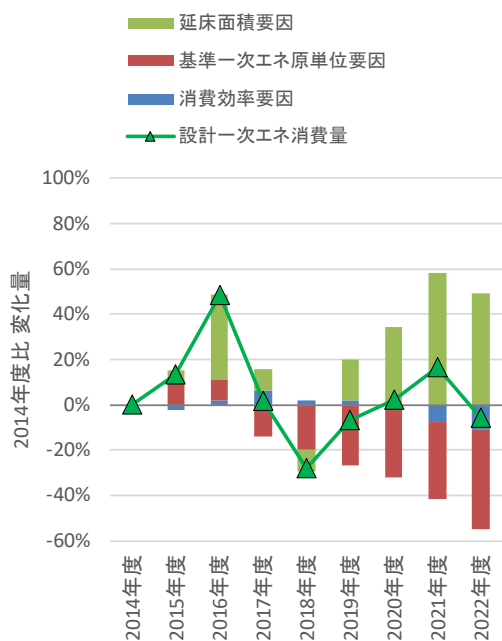
図Ⅲ-2-21 設計一次エネルギー消費量の2014年度比推移と増減要因分析
