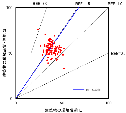
図 II-2-43 CASBEE 評価 BEE 値プロット図 (2021 年度 集合住宅)
