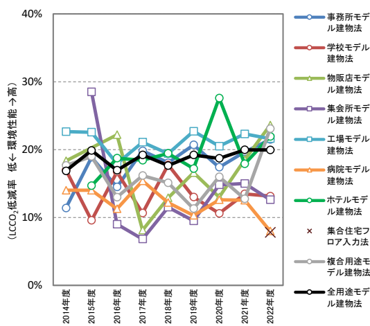
図II-2-77 CASBEE 評価における LCCO 2 低減率の建物用途別平均値 (モデル建物法等 簡易計算法 2014年度～2022年度) ※集合住宅は2022年度のみ
