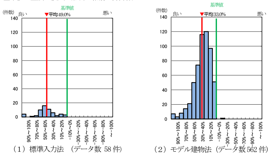
図 II-1-9 2022 年度 BEI 値 建物全体基準値からの削減
