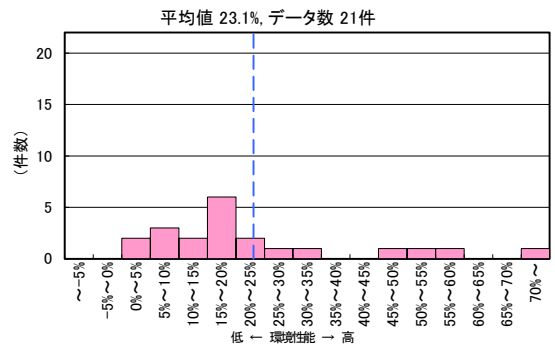
図Ⅱ-2-106 CASBEE 評価 LCCO 2 低減率の分布 (2022 年度 複合用途 モデル建物法)
