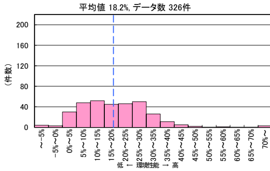
図 II-2-99 CASBEE 評価 LCCO 2 低減率の分布 (2008 年度～2021 年度 病院)
