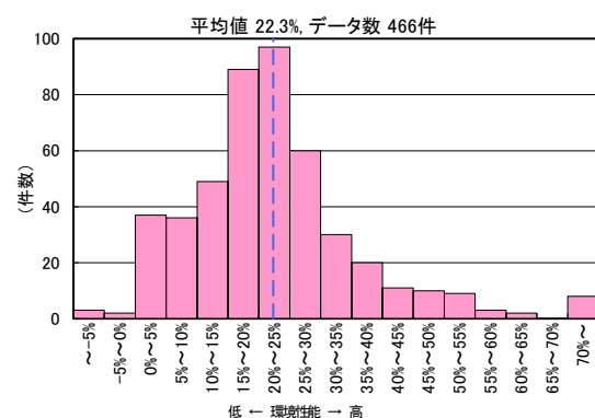
図Ⅱ-2-79 CASBEE評価 LCCO 2 低減率の分布 全用途 (2022年度)
