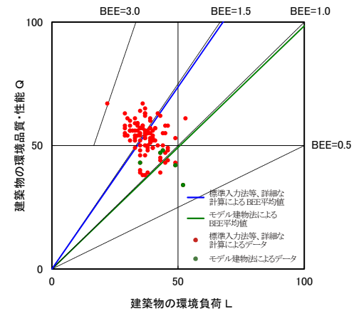
図 II-2-44 CASBEE 評価 BEE 値プロット図 (2022 年度 集合住宅)
