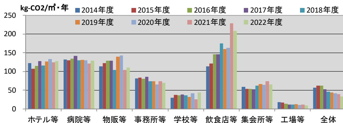
図Ⅲ-2-11 2014年度以降の建物用途毎 CO 2 排出原単位の推移
