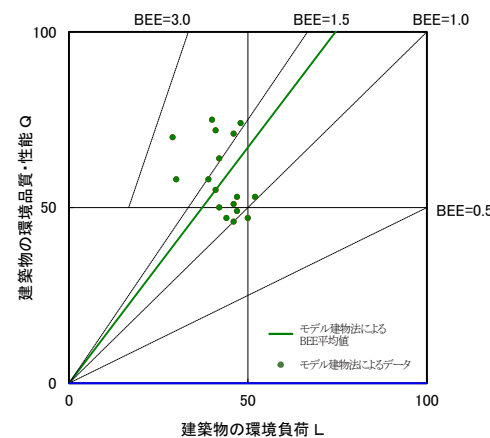
図 II-2-40 CASBEE 評価 BEE 値プロット図 (2022 年度 病院)
