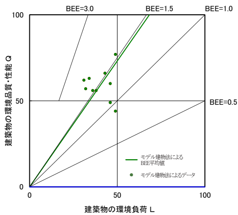
図 II-2-41 CASBEE 評価 BEE 値プロット図 (2021 年度 ホテル)
