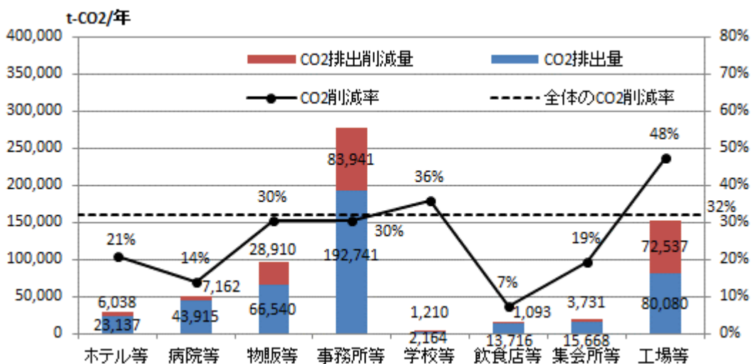
図Ⅲ-2-2 建物用途毎のCO 2 排出量とCO 2 排出削減量およびCO 2 削減率（昨年度調査）
