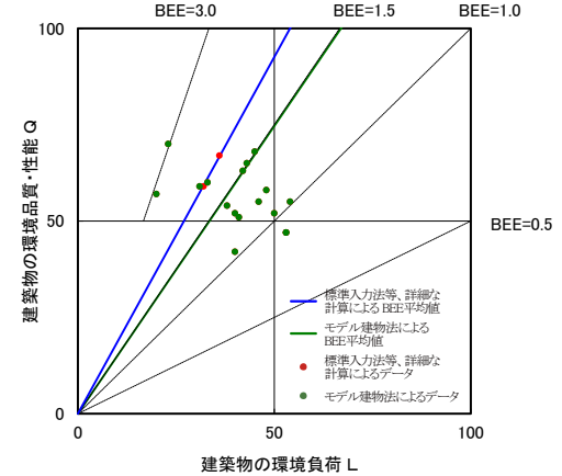
図II-2-33 CASBEE 評価 BEE 値プロット図 (2022 年度 物販店)
