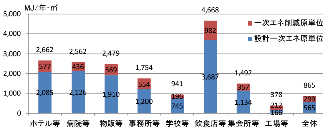
図Ⅲ-2-5 建物用途毎の設計一次エネ原単位と一次エネ削減原単位（今年度調査分）
