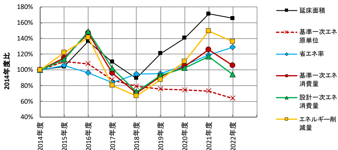
図Ⅲ-2-17 延床面積、基準一次エネ原単位、省エネ率と一次エネルギー消費関連量の2014年度比推移 ※ グラフ中の年度は届出年度。BEI評価となった2014年度を基準年とした。2017年度に適合義務化が開始。
