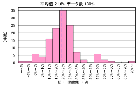
図 II-2-98 CASBEE 評価 LCCO 2 低減率の分布 (2022 年度 工場 モデル建物法)
