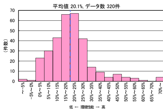
図 II-2-83 CASBEE 評価 LCCO 2 低減率の分布 2022 度 非住宅 (モデル建物法)
