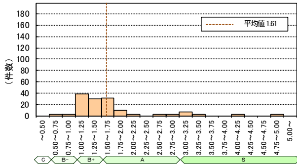
図II-2-65 CASBEE 評価 BEE 値の分布 (2017 年度 標準入力法等、詳細計算法)
