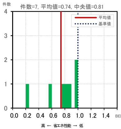
図Ⅱ-1-31 BEI の分布 (飲食店等 モデル建物法)
