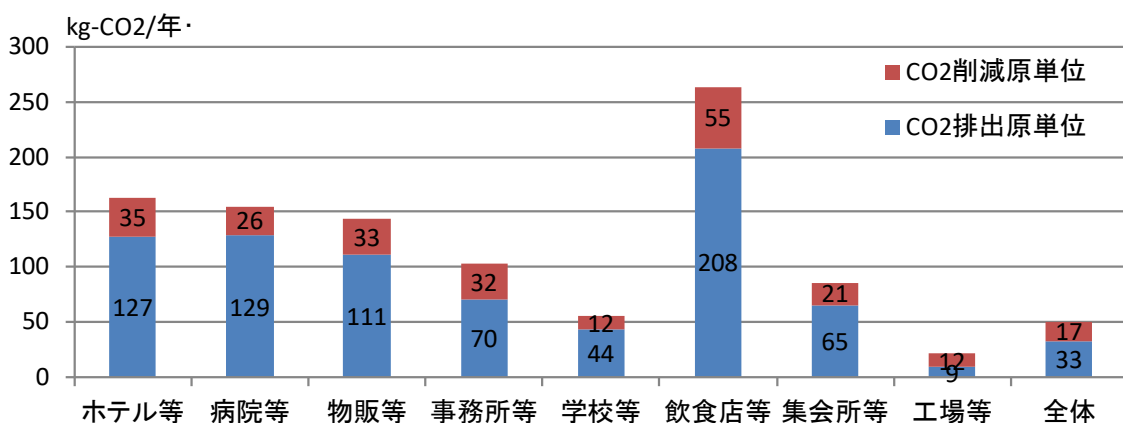
図Ⅲ-2-7 建物用途毎のCO 2 排出原単位とCO 2 削減原単位（今年度調査分）
