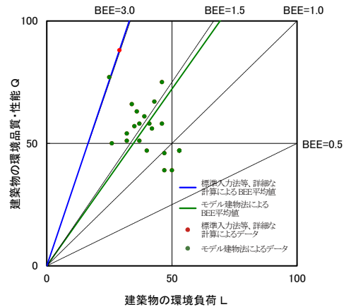
図 II-2-46 CASBEE 評価 BEE 値プロット図 (2022 年度 複合用途)
