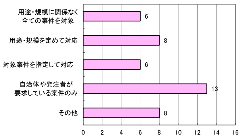
図 I-1-1 CASBEE による評価を行う対象案件 (30 社)
