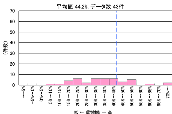
図 II-2-82 CASBEE 評価 LCCO 2 低減率の分布 2022 度 非住宅 (標準入力法等)
