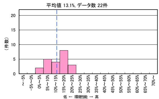
図 II-2-89 CASBEE 評価 LCCO 2 低減率の分布 (2022 年度 学校 モデル建物法)
