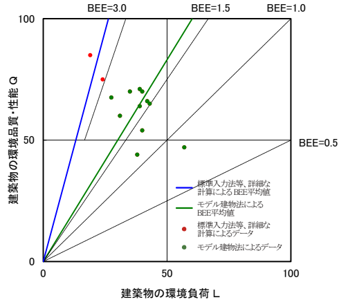
図 II-2-36 CASBEE 評価 BEE 値プロット図 (2022 年度 集会所)
