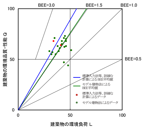
図 II-2-45 CASBEE 評価 BEE 値プロット図 (2021 年度 複合用途)
