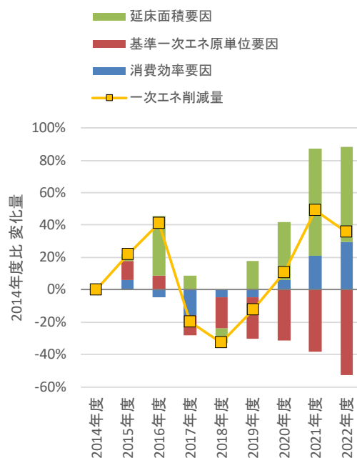
図Ⅲ-2-22 一次エネルギー削減量の2014年度比推移と増減要因分析
