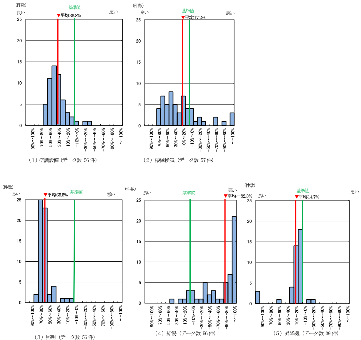
図Ⅱ-1-11 2022 年度 標準入力法 各設備機器 基準値からの削減率
