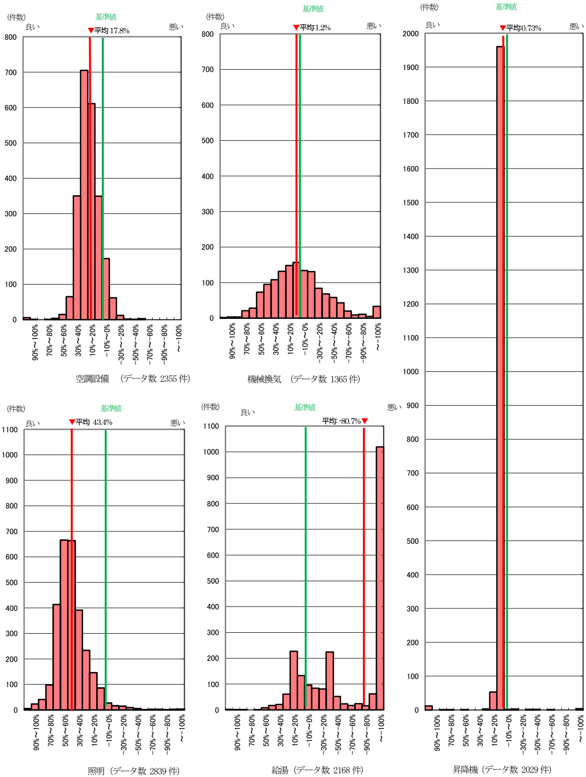
図Ⅱ-I-14 2013～2022 年度 モデル建物法 各設備機器 基準値からの削減率
