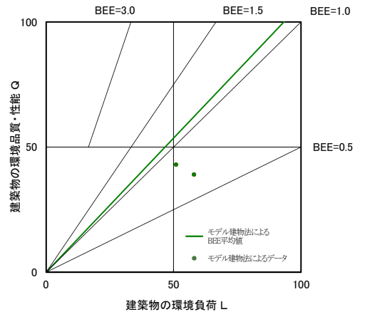
図II-2-34 CASBEE 評価 BEE 値プロット図 (2022 年度 飲食店)
