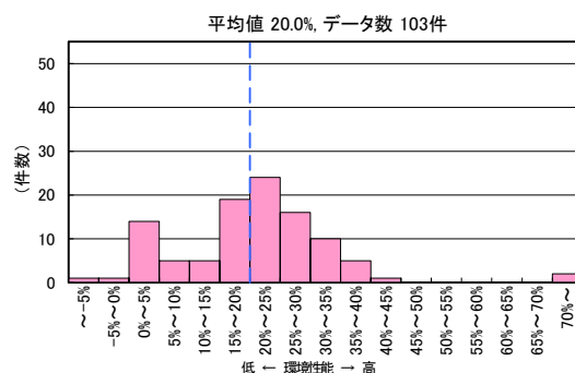
図 II-2-81 CASBEE 評価 LCCO 2 低減率の分布 (2022 年度 集合住宅)
