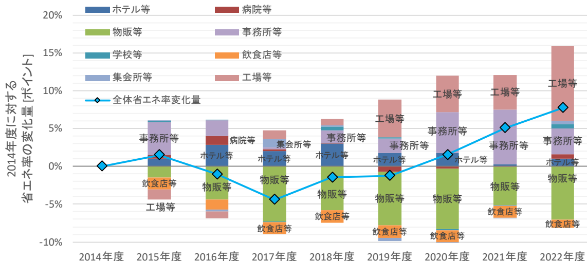
図Ⅲ-2-25 全体の省エネ率の 2014 年度に対する変化量とその建物用途ごとの変化量
