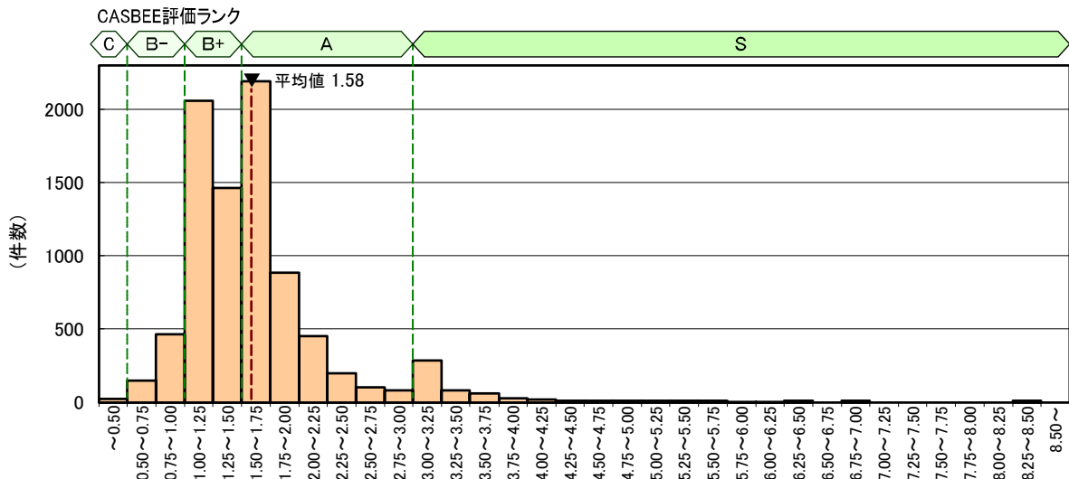
図II-2-48 CASBEE 評価 BEE 値の分布 (2004～2022 年度データ 全用途)
