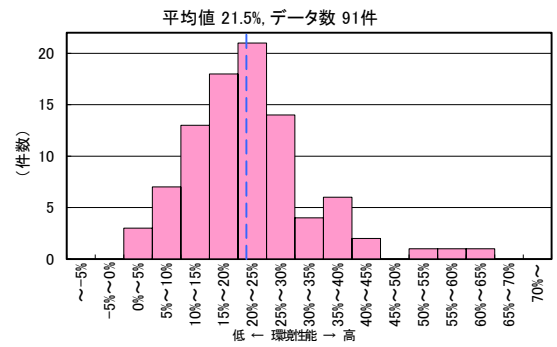
図 II-2-86 CASBEE 評価 LCCO 2 低減率の分布 (2022 年度 事務所 モデル建物法)
