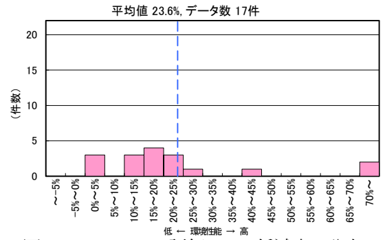
図 II-2-92 CASBEE 評価 LCCO 2 低減率の分布 (2022 年度 物販店 モデル建物法)
