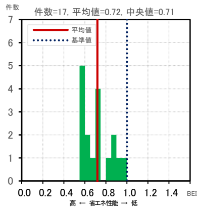
図II-1-35 BEIの分布 (ホテル モデル建物法)
