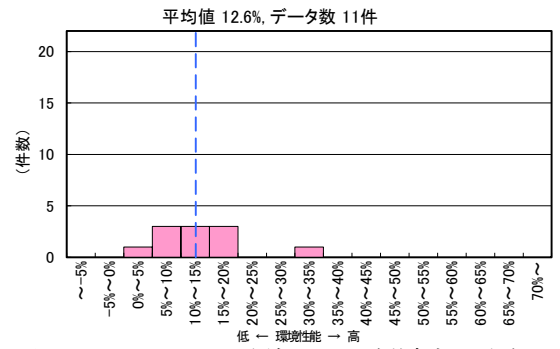
図 II-2-95 CASBEE 評価 LCCO 2 低減率の分布 (2022 年度 集会所 モデル建物法)
