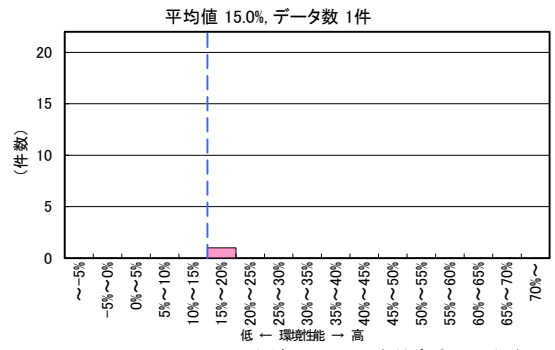
図Ⅱ-2-105 CASBEE 評価 LCCO 2 低減率の分布 (2022 年度 複合用途 標準入力法等)
