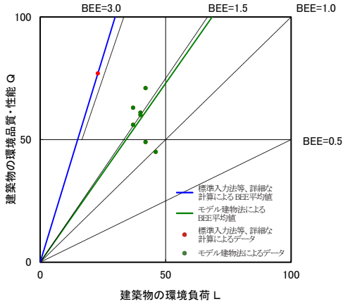
図II-2-30 CASBEE 評価 BEE 値プロット図 (2021 年度 学校)
