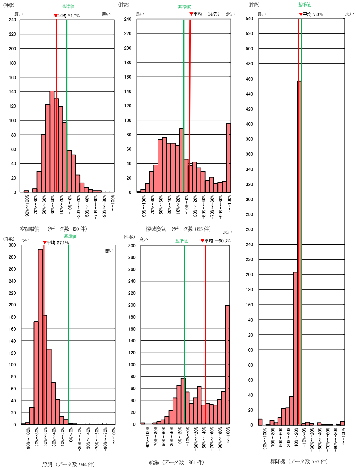
図Ⅱ-1-13 2013～2022 年度 標準入力法 各設備機器 基準値からの削減率
