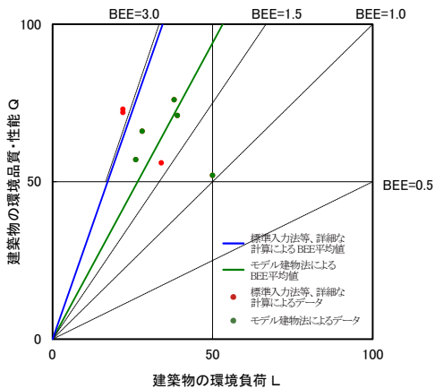
図 II-2-35 CASBEE 評価 BEE 値プロット図 (2021 年度 集会所)
