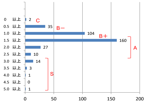
図Ⅱ-2-103 BEE の度数分布 (2022 年度) (N=357)
