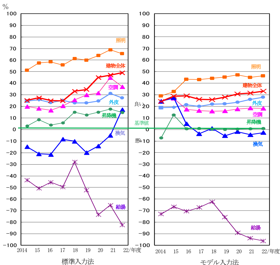
図Ⅱ-1-6 各指標の基準値に対する削減率平均値の推移（2014年度～2022年度）
