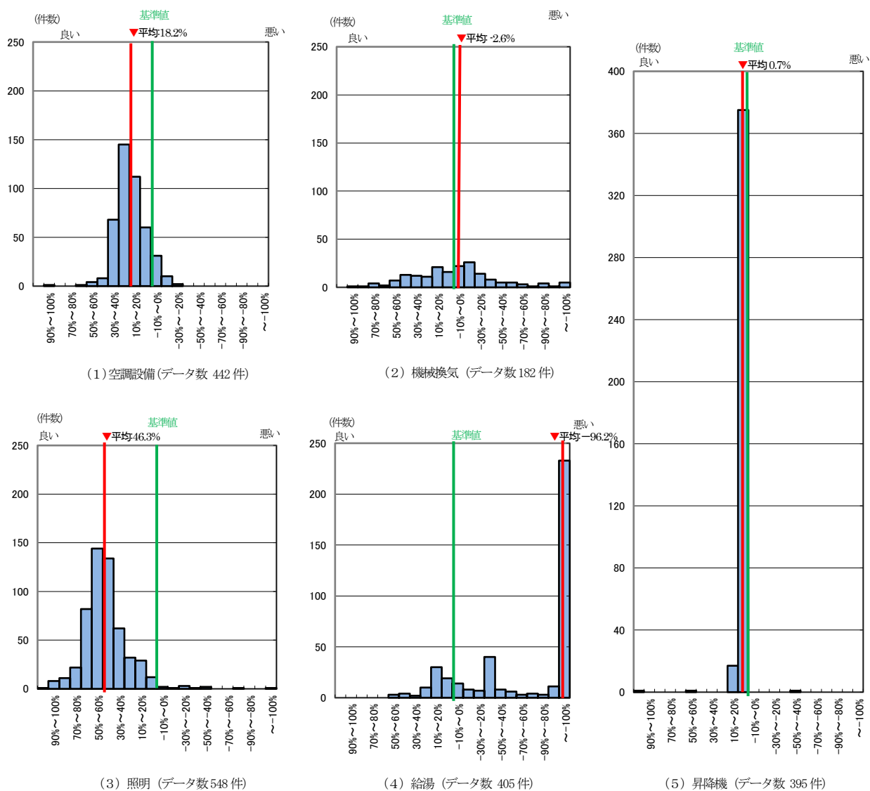
図Ⅱ-1-12 2022年度 モデル建物法 各設備機器 基準値からの削減率
