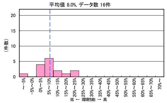
図 II-2-101 CASBEE 評価 LCCO 2 低減率の分布 (2022 年度 病院 モデル建物法)
