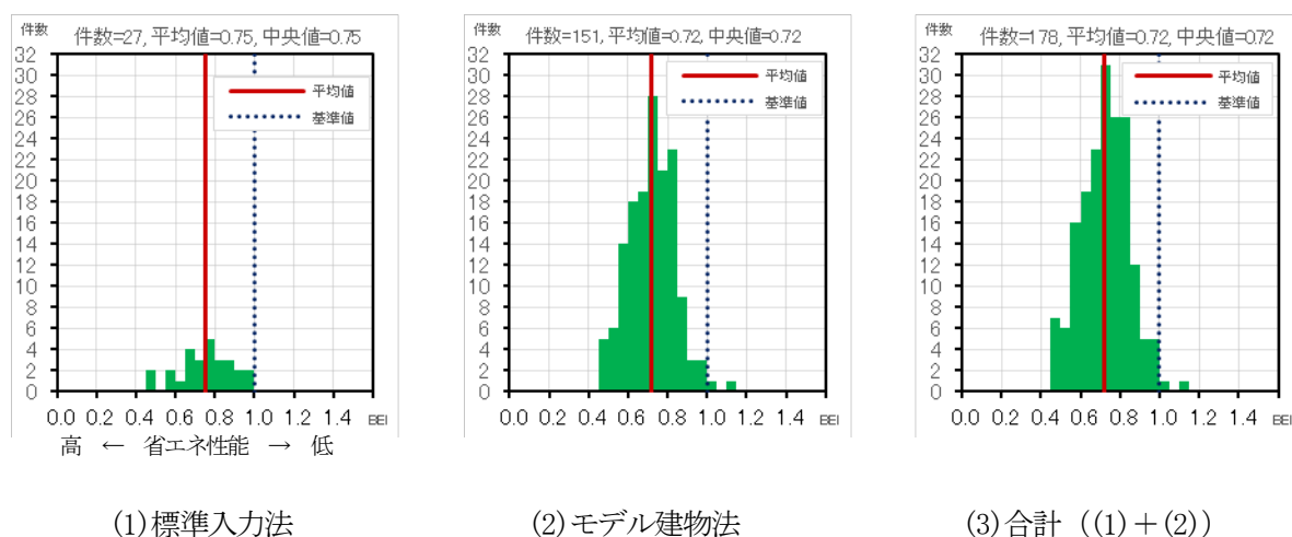
図Ⅱ-1-16 BPI の分布 (事務所)
