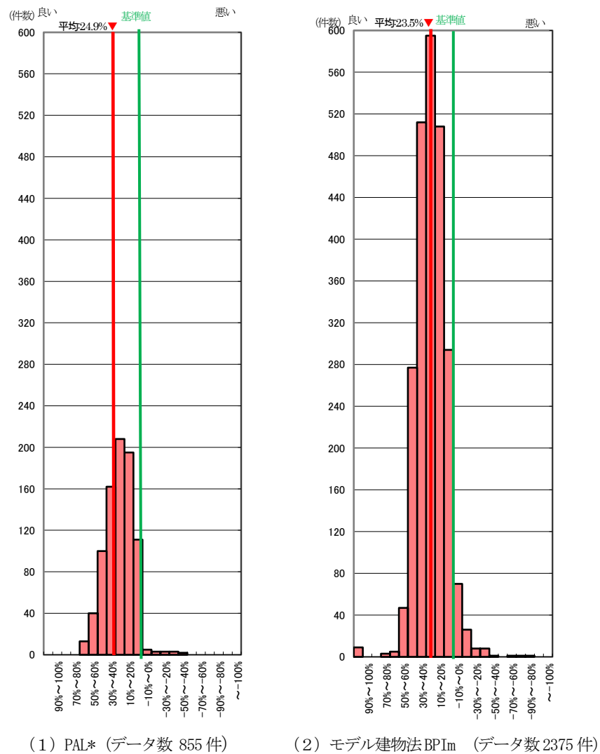
図 II-1-8 2013～2022 年度 外皮性能の基準値からの削減率
