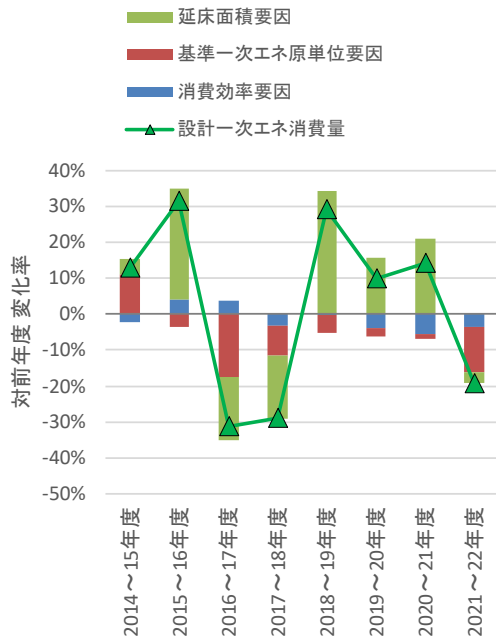
図Ⅲ-2-23 設計一次エネルギー消費量の 前年度比推移と増減要因分析
