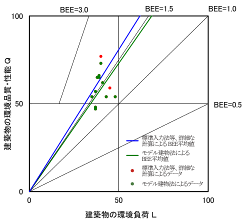
図 II-2-39 CASBEE 評価 BEE 値プロット図 (2021 年度 病院)
