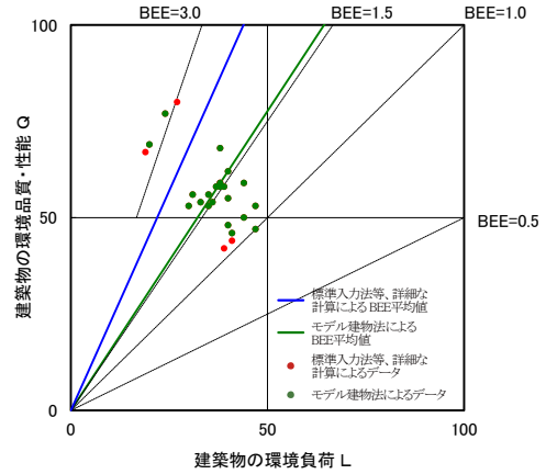
図II-2-31 CASBEE 評価 BEE 値プロット図 (2022 年度 学校)
