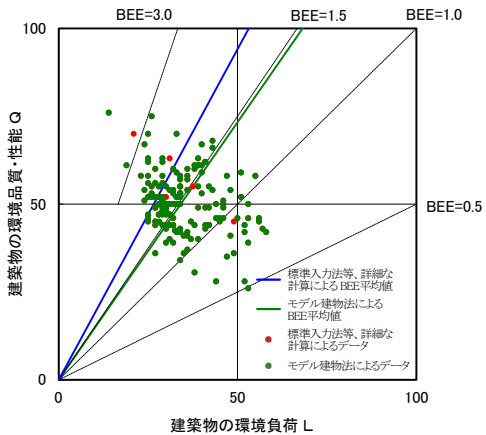
図 II-2-37 CASBEE 評価 BEE 値プロット図 (2021 年度 工場)
