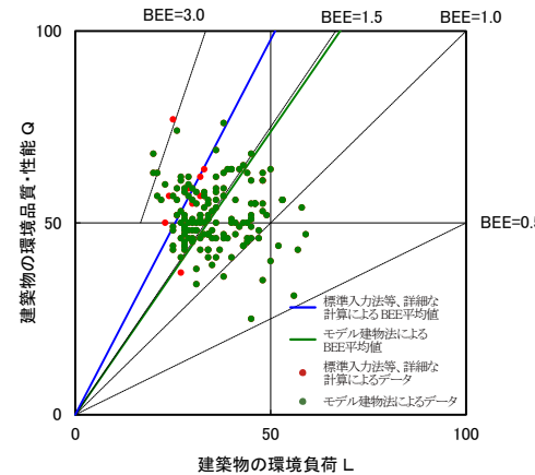
図 II-2-38 CASBEE 評価 BEE 値プロット図 (2022 年度 工場)
