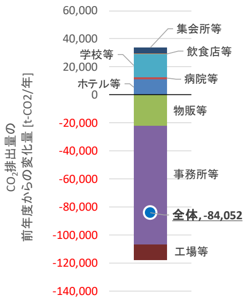
図Ⅲ-2-3 CO 2 排出量の前年度からの変化量
