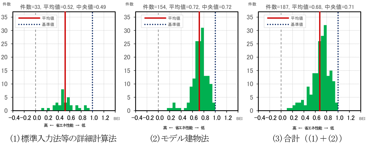
図Ⅱ-1-28 BEIの分布 (事務所)
