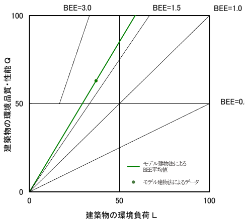
図II-2-34 CASBEE 評価 BEE 値プロット図 (2021 年度 飲食店)
