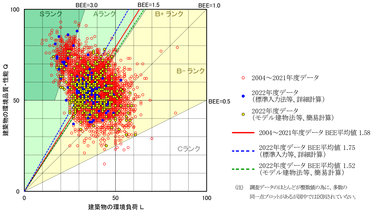
図II-2-47 CASBEE 評価 BEE 値プロット図 (2004～2022 年度データ 全用途)
