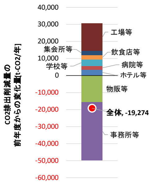
図Ⅲ-2-4 CO 2 排出削減量の前年度からの変化量
