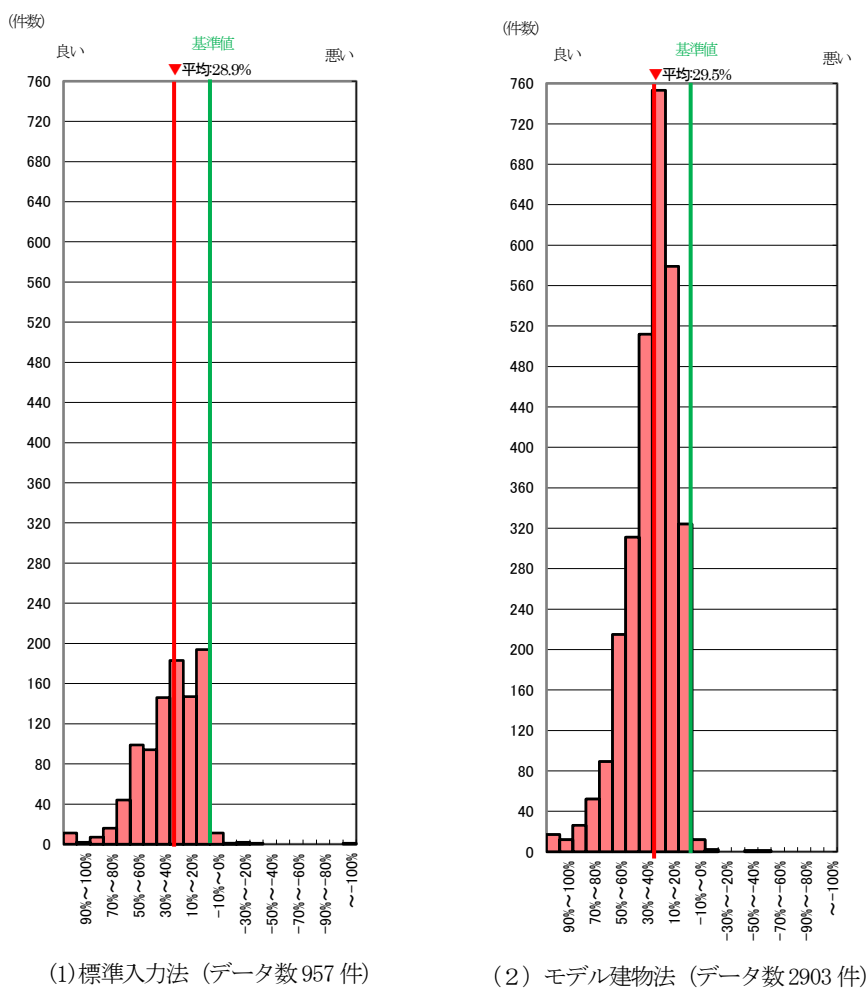
図 II-1-10 2013～2022 年度 BEI 値 建物全体基準値からの削減
