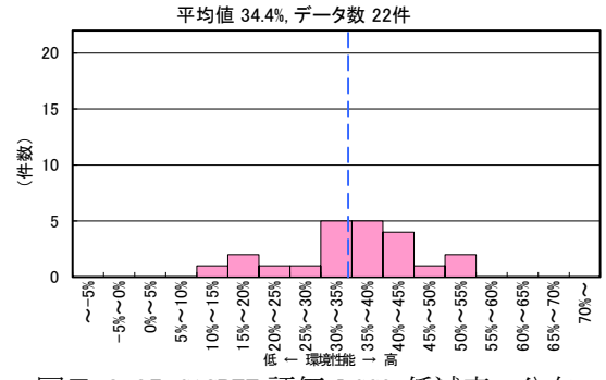
図 II-2-85 CASBEE 評価 LCCO 2 低減率の分布 (2022 年度 事務所 標準入力法等)
