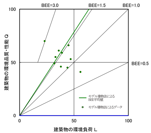
図 II-2-42 CASBEE 評価 BEE 値プロット図 (2022 年度 ホテル)
