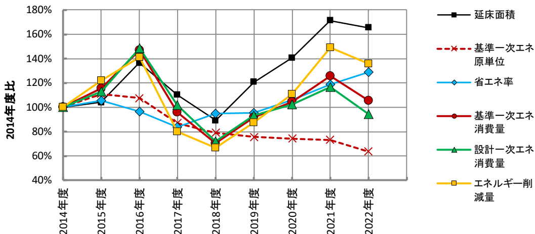
(再掲) 図Ⅲ-2-17 延床面積、基準一次エネ原単位、省エネ率と一次エネルギー消費関連量の推移
