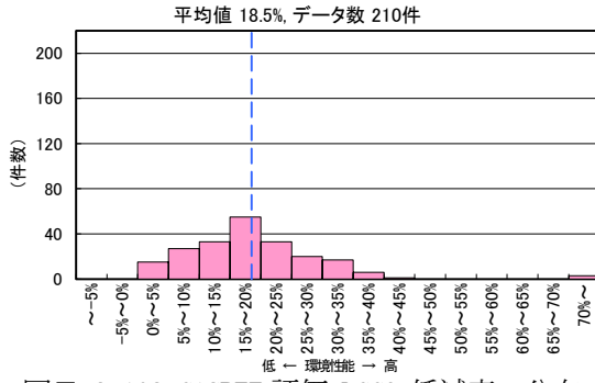
図Ⅱ-2-102 CASBEE 評価 LCCO 2 低減率の分布 (2008 年度～2021 年度 ホテル)
