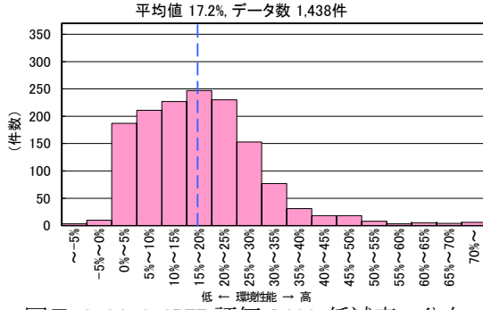
図 II-2-96 CASBEE 評価 LCCO 2 低減率の分布 (2008 年度～2021 年度 工場)
