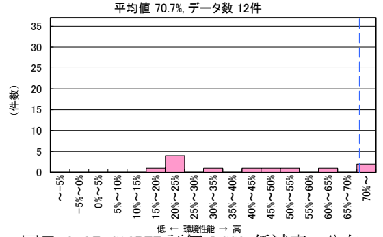
図 II-2-97 CASBEE 評価 LCCO 2 低減率の分布 (2022 年度 工場 標準入力法等)
