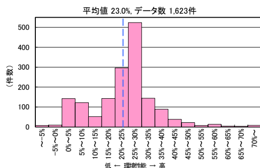
図 II-2-80 CASBEE 評価 LCCO 2 低減率の分布 (2008 年度～2021 年度 集合住宅)
