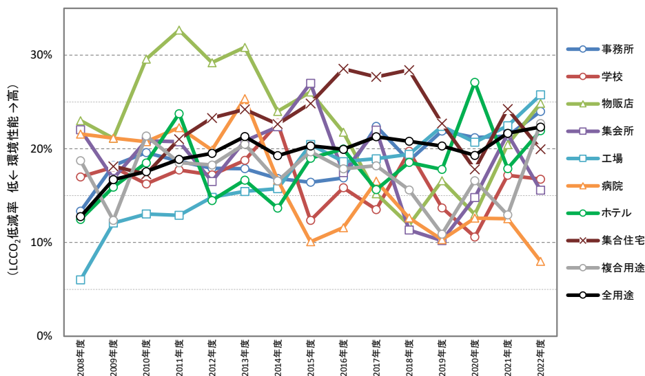
図II-2-75 CASBEE 評価における LCCO 2 低減率の建物用途別平均値 (2008年度～2022年度データ)
