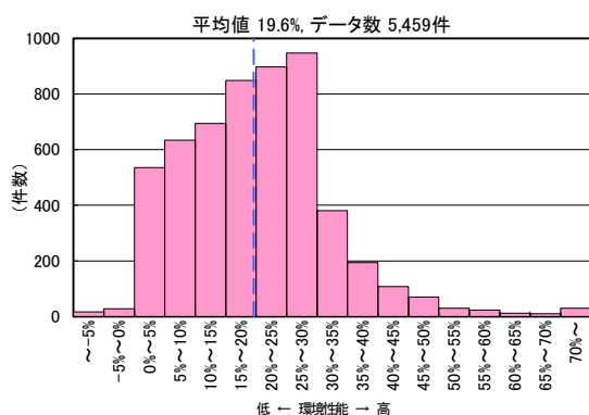
図Ⅱ-2-78 CASBEE評価 LCCO 2 低減率の分布 全用途 (2008年度～2021年度)
