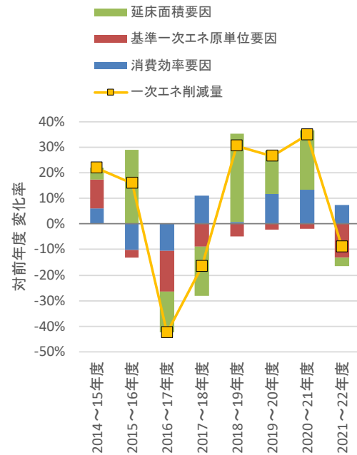
図Ⅲ-2-24 一次エネルギー削減量の 前年度比推移と増減要因分析
