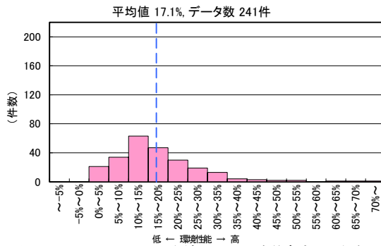
図 II-2-87 CASBEE 評価 LCCO 2 低減率の分布 (2008 年度～2021 年度 学校)
