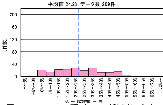
図 II-2-90 CASBEE 評価 LCCO 2 低減率の分布 (2008 年度～2021 年度 物販店)
