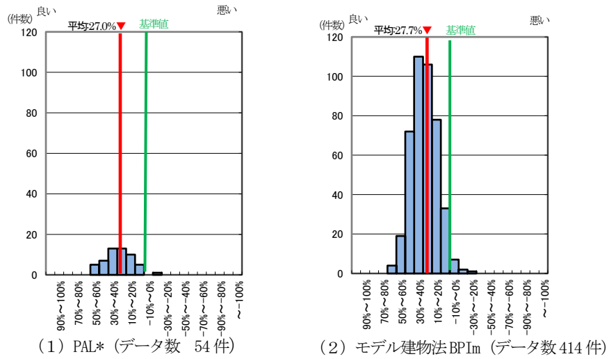
図 II-1-7 2022 年度 外皮性能の基準値からの削減率
