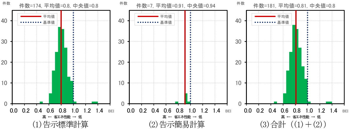
図Ⅱ-1-27 BEIの分布 (集合住宅)
