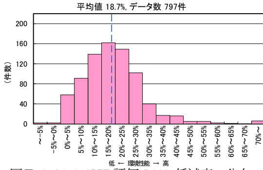
図 II-2-84 CASBEE 評価 LCCO 2 低減率の分布 (2008 年度～2021 年度 事務所)
