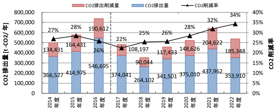
図Ⅲ-2-9 2014年度以降のCO 2 排出量とCO 2 排出削減量、CO 2 削減率の推移
