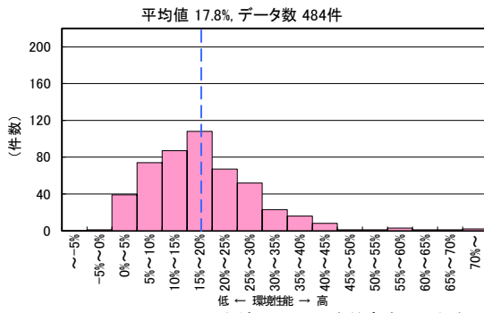
図Ⅱ-2-104 CASBEE 評価 LCCO 2 低減率の分布 (2008 年度～2021 年度 複合用途)
