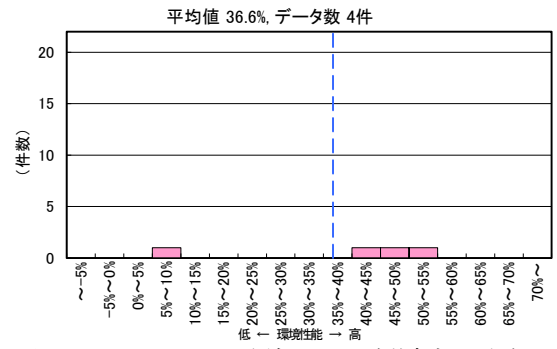
図 II-2-88 CASBEE 評価 LCCO 2 低減率の分布 (2022 年度 学校 標準入力法等)
