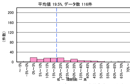
図 II-2-93 CASBEE 評価 LCCO 2 低減率の分布 (2008 年度～2021 年度 集会所)
