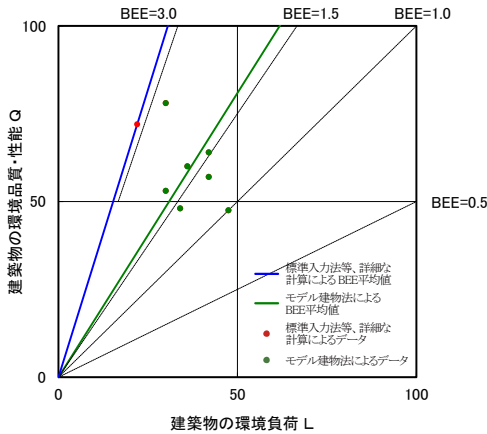
図II-2-32 CASBEE 評価 BEE 値プロット図 (2021 年度 物販店)
