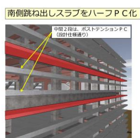
南側の跳ね出しスラブをハーフPC化した。大梁底に取り付く形となっている。
