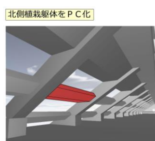
北側に1フロア3段ある植栽躯体をPC化した。植栽躯体とは、部材としては「大梁」である。
