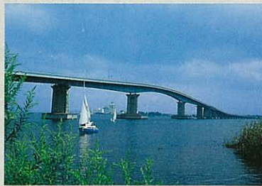
●表紙: 琵琶湖大橋 滋賀県中央部に県の6分の1の面積をもって広がる日本一の大湖。そして、日本の歴史と文化のふるさとである琵琶湖。その観光の中心である湖東の守山と湖西の堅田間1,350mを結ぶ道路橋として、1964年に完成した。主径間長140m 主径間の下は定期遊覧船の航行に支障のないよう、水面上20mの空間をもたせている。また、水深が深いため1.2mもの大口径鋼管杭を用いている。
